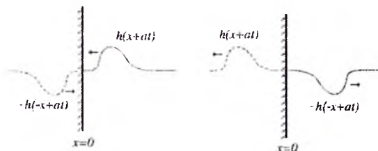
V.2-rasmi: Bir uchi mahkamlangan tor bo'yicha to'liqin tarqalishi
