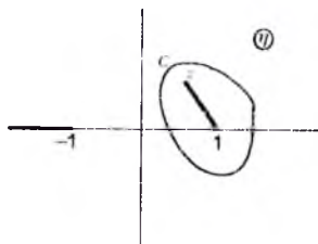
I.2-rasm: Schläfli integrali uchun kontur
