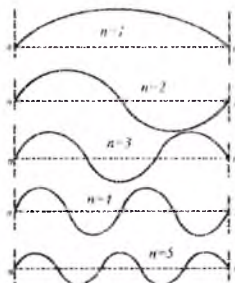
VI.1-rasm: Turg'un to'lqinlar
