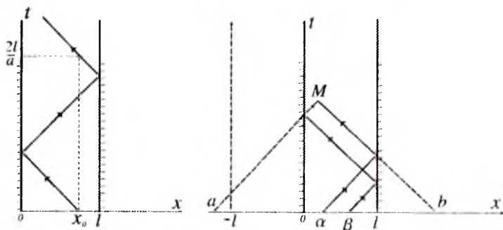
V.4-rasin: Ikki uchi mahkamlangan tor
