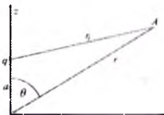
1.1-rasim: z = a o'qida joylashgan zaryad
