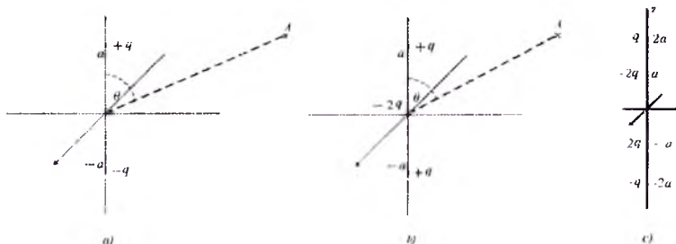
1.4-rasm: Zaryadlar sistemalari
