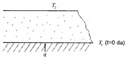
VI.2-rasim: Yer sirtining sovishi
