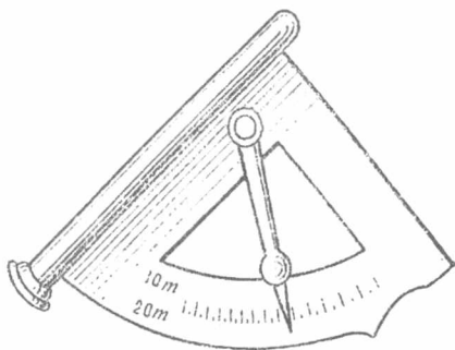
16-rasm. Daraxt balandligini Makarov ish qurolida o'lchash.
