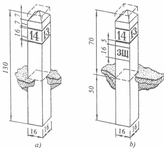
39-rasm. Kvartal stolbalarining tuzilishi.
