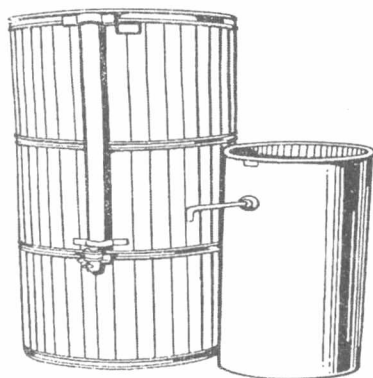
24-rasm. Ksilometrlar: chapda — o'zgaruvchan suv sathi bilan; o'ngda — o'zgarmas suv sathi bilan.
