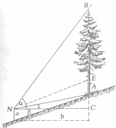
16-rasm. Daraxt balandligini Makarov ish qurolida o'lchash.
