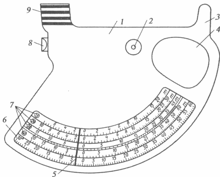
7-rasm. Blyume-Leyssanining daraxtlar balandlik o'lchagichi.
