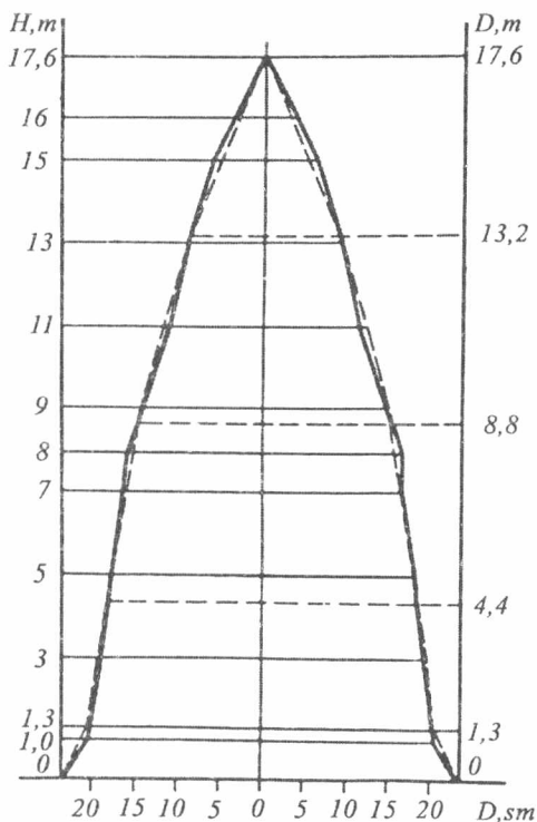
35-rasm. Daraxt tanasi shakl koefitsiyentini aniqlashda o'lchab olinadigan asosiy diametrilar.
