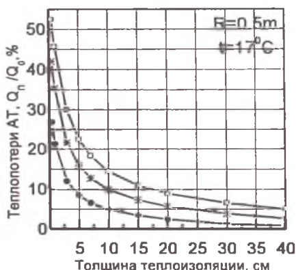
Рисунок 2 - Тепловые потери водяного двухслойного шарового аккумулятора тепла с радиусом 0.5 м, в зависимости от толщины теплоизоляции при различных сроках хранения воды: 24ч - ●, 48ч - ×, 72ч - □.
