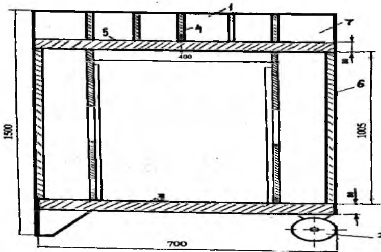
Рисунок 4 - Конструктивная схема станины переносного камнекольного пресса ПКП-300
