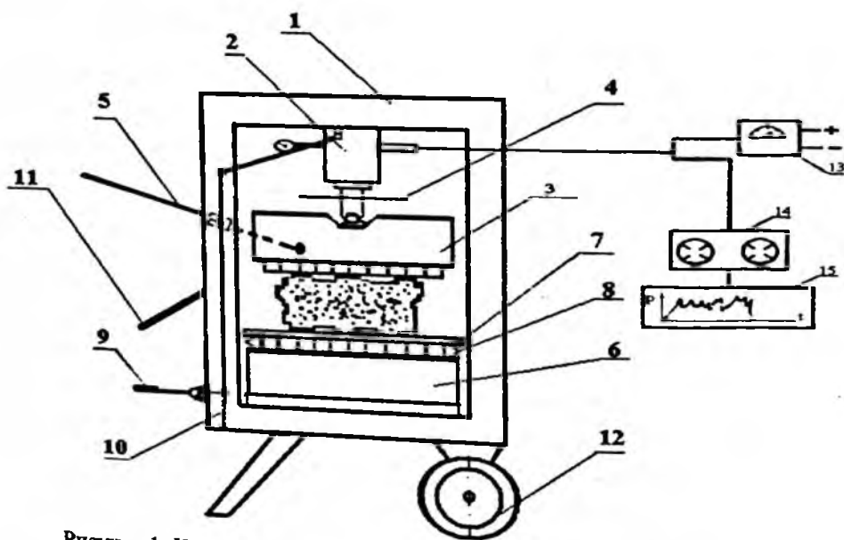
Рисунок 1- Конструктивная схема переносного камнекольного пресса ПКП-300: 1-гидравлический домкрат; 2 – станина; 3- верхний рабочий орган; 4 – ручка для поворота винта; 5 – рычаг для подъема рабочего органа; 6 – нижний рабочий орган; 7 – рабочий стол; 8 – упругие пружины; 9-ножной педаль для качания домкрата; 10 – упругая пружина для возврата педали; 11- Рукоятка для переноса; 12 – колесо для передвижения; 13 – источник постоянного тока типа «Агат»; 14 – магнитофон «Брюль и Кьер»; 15 – самопишущее устройство.
