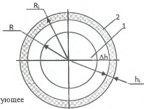
Рисунок 1 - Схема двухслойного шарового аккумулятора тепла
