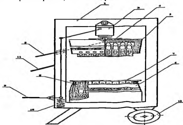
Рисунок 3- Конструкция переносного камнекольного прессы ПКП-300
