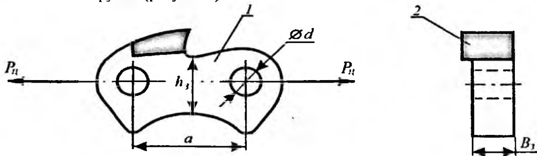
1 - звено режущей цепи; 2 - твердосплавный резец. Рисунок 1 - Режущее звено цепного рабочего органа
