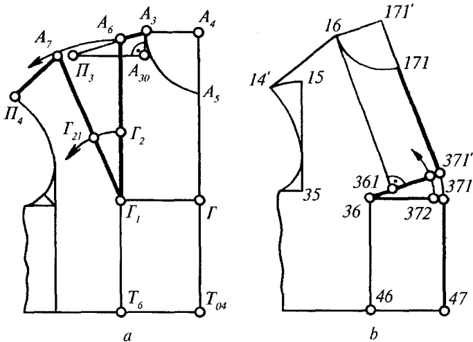
2.16-rasm. Yuqori vitachkani qurish: a — ЦНИИШП uslubi; b — ЕМКО.
