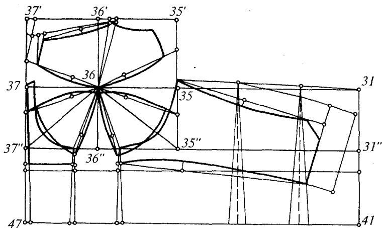
2.67-rasm. O'yalsimon o'tqazma kosali byustgaiter detallarining chizmasi.
