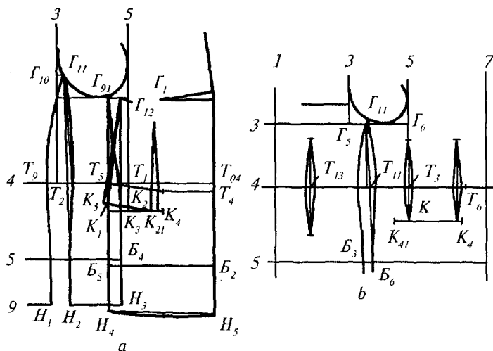
2.20-rasm. ЦНИИШП uslubii bo'yicha chizmada yon, bel, etak chiziqlarini, vitachkalarni va yon cho'ntaklar chiziqlarini qurish: a — pidjakda; b — ayollar paltosida.
