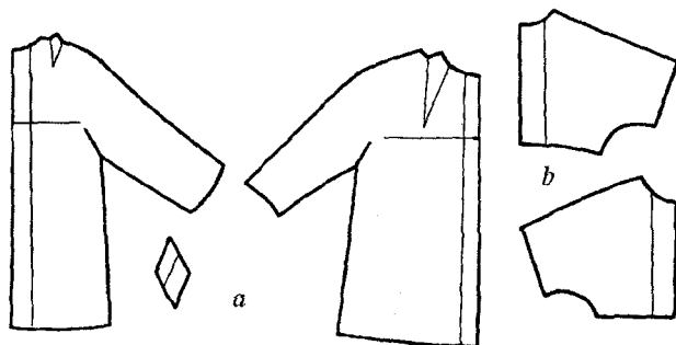
1.24-rasm. Yaxlit bichilgan yengli kiyimning asosiy detallari.
