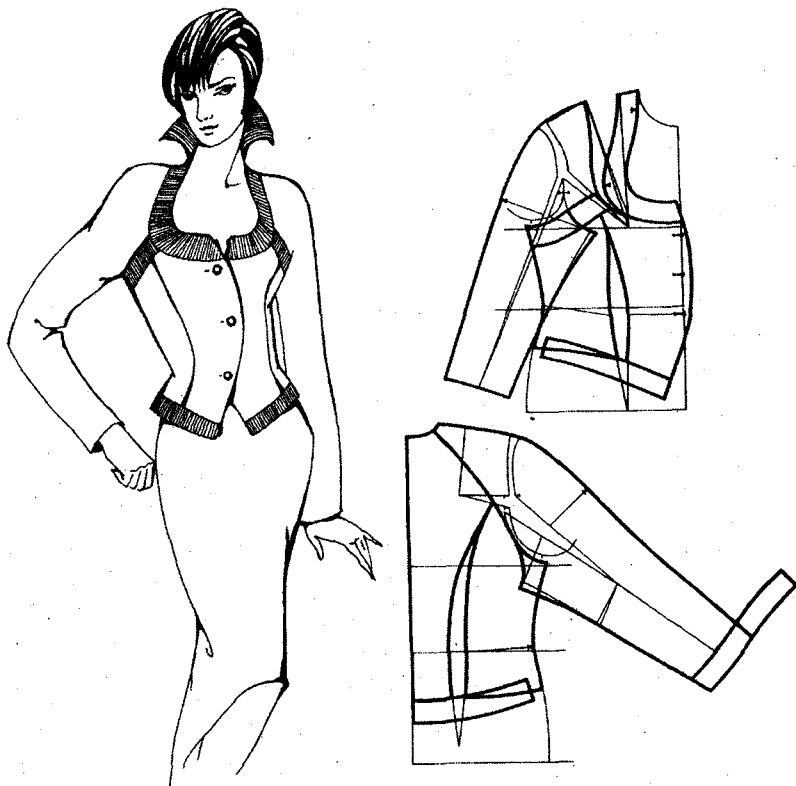
3.31-rasm. Yengi kombinatsiyalashtirilgan bichimli jaketning konstruksiyasi.
