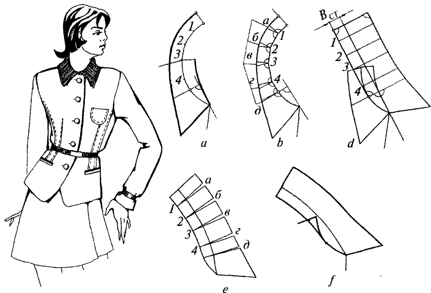
3.18-rasm. Qaytarma yoqani qurish sxemasi:
