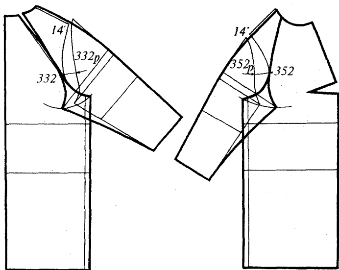
3.25-rasm. Shakli yumshoq reglan bichimli yengning konstruktiv ko'rinishi.
