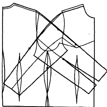
3.33-rasm (a, b). Yaxlit bichilgan yengli va qirqma yon bo'lakli konstruksiyani qurish.
