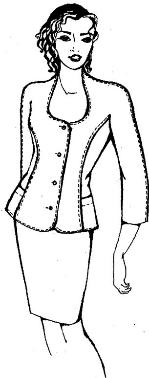
3.32-rasm. O‘mizdan chiqqan burma chokli yaxlit bichilgan yangli jaketning konstruksiyasi.
