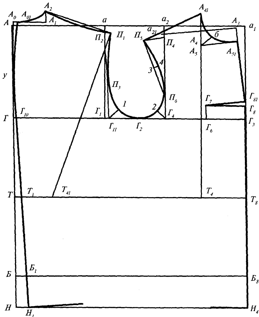
I.4.2.1-rasm. Erkaklar yelka kiyimi asosiy konstruksiyasi
