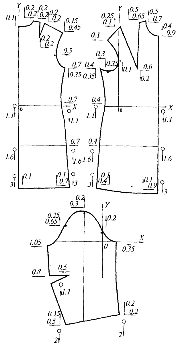
5.6-rasm. Ayollar kiyimiga doir asosiy detallar razmerlar bo'yicha (X strekkali belgilangan) bo'ylar bo'yicha (Y aylanalni strelka bilan belgilangan) gradatsiyasining sxemasi.
