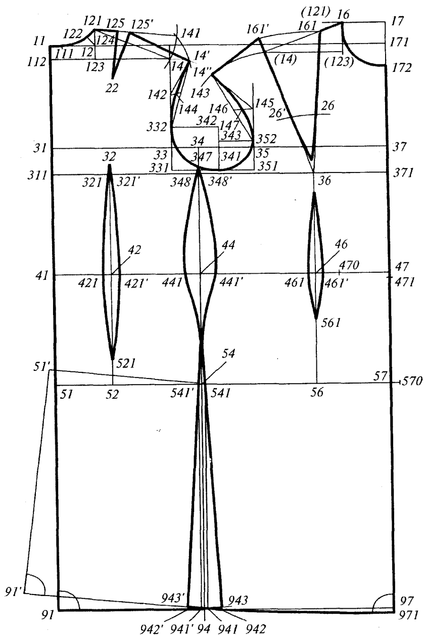
2.26-rasm. МГУТД uslubi bo'yicha nim yopishgan siluetti ayollar ko'ylagining konstruksiyasi.
