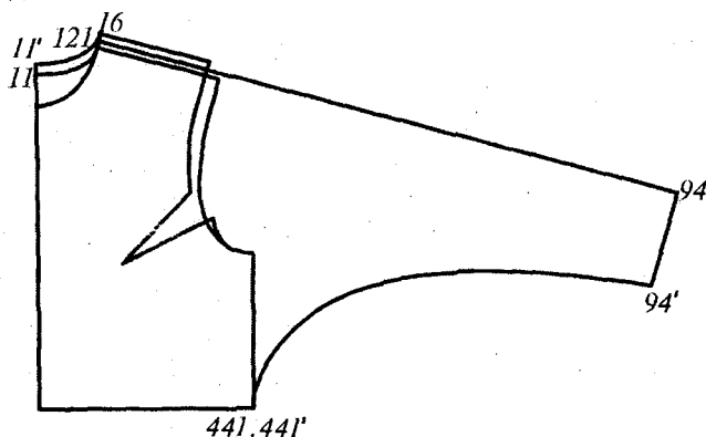
3.36-rasm. Yaxlit bichilgan yengli yumshoq shaklli trikotaj buyum konstruksiyasi.
