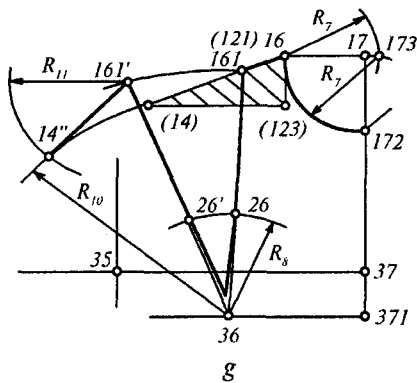
2.25-rasm. Yuqori konstruktiv chiziqlari qurish.
