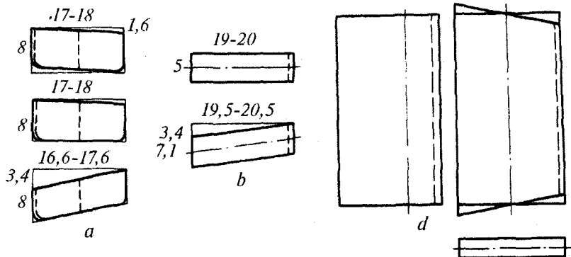
3.45-rasm. Erkaklar pidjagi yon cho'ntagining unifikatsiyalangan detallari.
