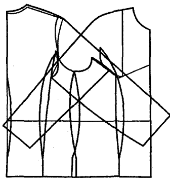
3.33-rasm (a, b). Yaxlit bichilgan yengli va qirqma yon bo'lakli konstruksiyani qurish.
