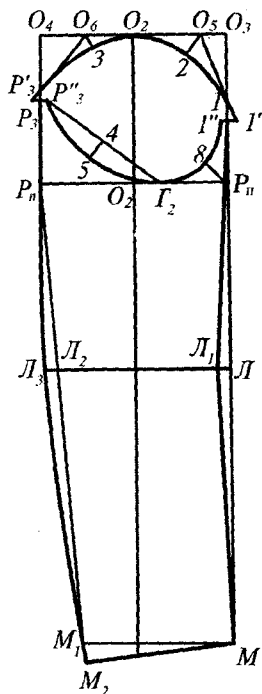
I.4.1.2-rasm. O'tqazma yeng asosiy konstruksiyasi.
