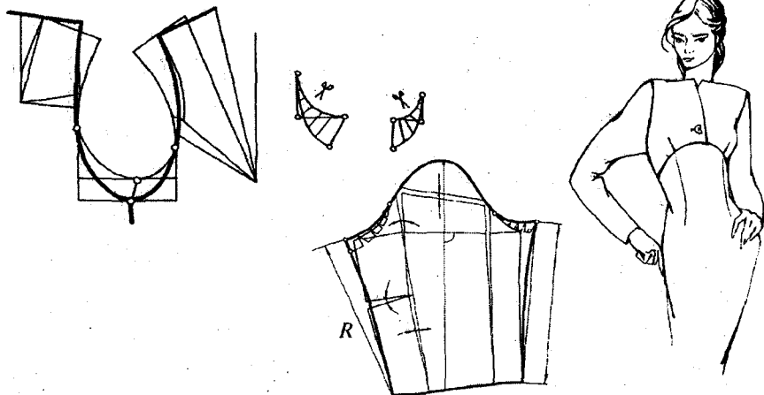
3.21-rasm. Yelka yostiqli va chuqurlashtirilgan o‘mizli ko‘ylakning bir chokli o‘tqazma yengini modellashtirish sxemasi.
