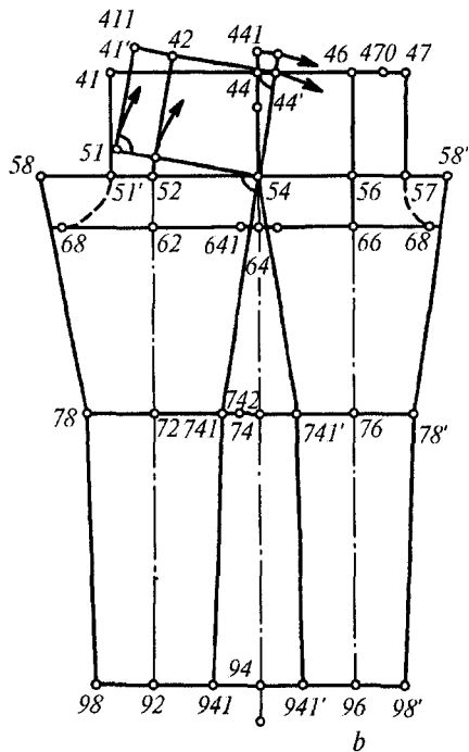
2.47-rasm. Erkaklar shimining konstruksiyasi: a — ЦНИИШП uslubi bo'yicha; b — ЕМКО.
