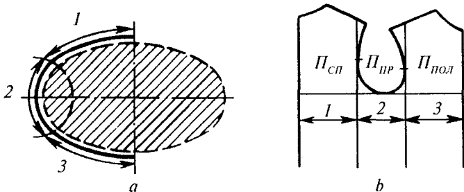
1.17-rasm. Kiyimda (a) va chizmada (b) konstruksiyaning asosiy uchastkalari aro ko'krak aylanasiga qo'shimchani taqsimlanishi.
