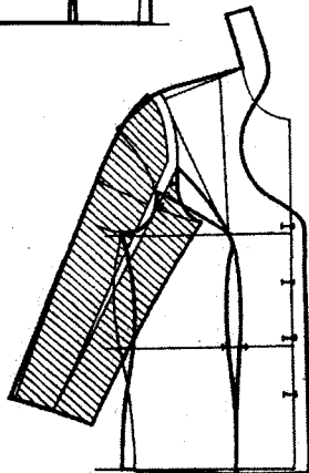
3.32-rasm. O‘mizdan chiqqan burma chokli yaxlit bichilgan yangli jaketning konstruksiyasi.
