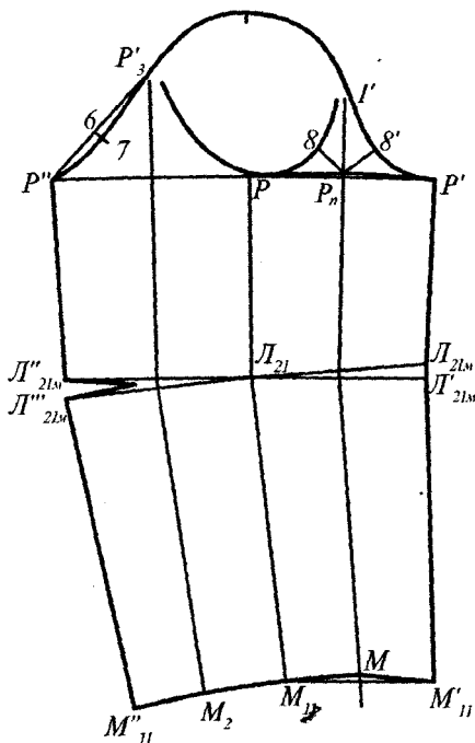
I.4.1.2-rasm. O'tqazma yeng asosiy konstruksiyasi.
