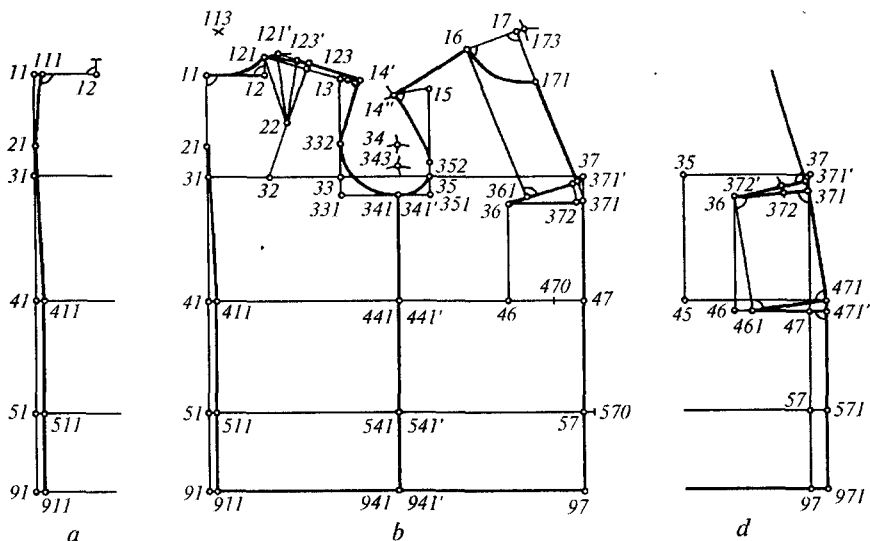
2.23-rasm. EMKO uslubi bo'yicha tananing yuqori qismiga mo'ljallangan chizma.
