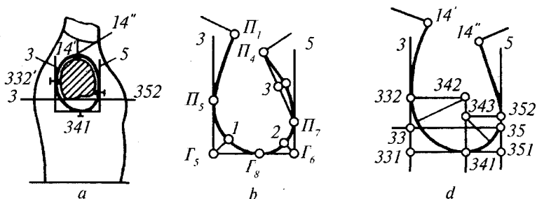
2.17-rasm. O'miz chizig'ining buyumda joylanishi (a) va chizmada qurish usullari: b — ЦНИИШП uslub; d — EMKO.
