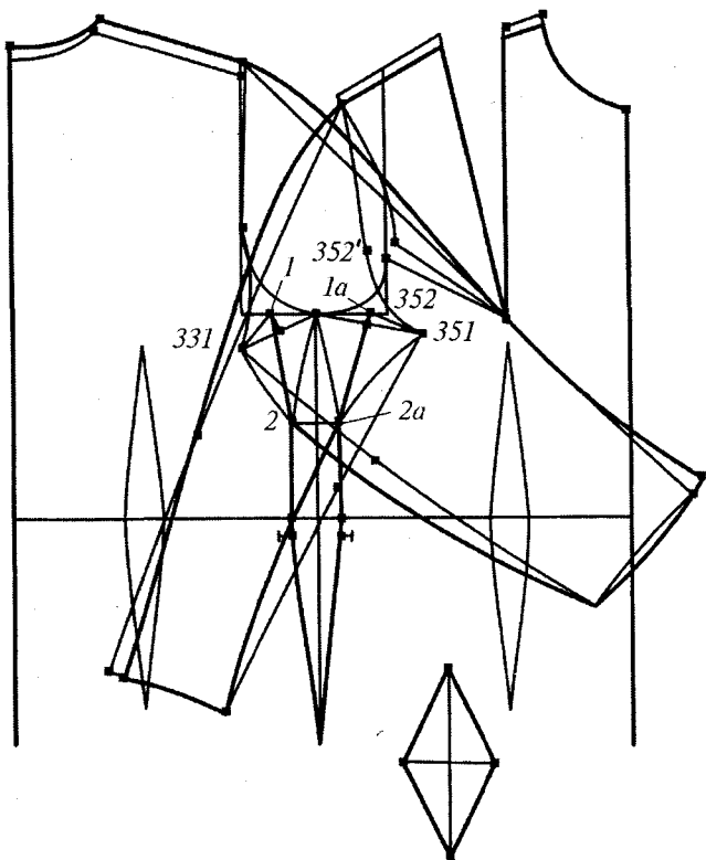
3.37-rasm. Dastlabki tana va yeng detallari asosida qurilgan xishtakli yaxlit bichilgan yangli buyum konstruksiyasi.
