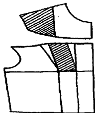
3.2-rasm. Ko'krak markazidan o'tgan bo'linish chiziqlarini qurish va ularning markazdan surilishi.
