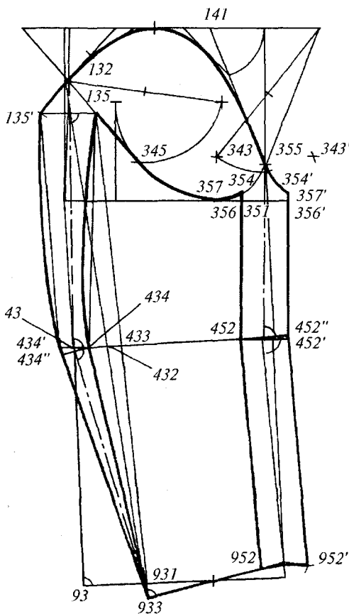
2.35-rasm. Nim yopishgan siluetti palto ikki chokli yengining modelga xos konstruksiyasi.
