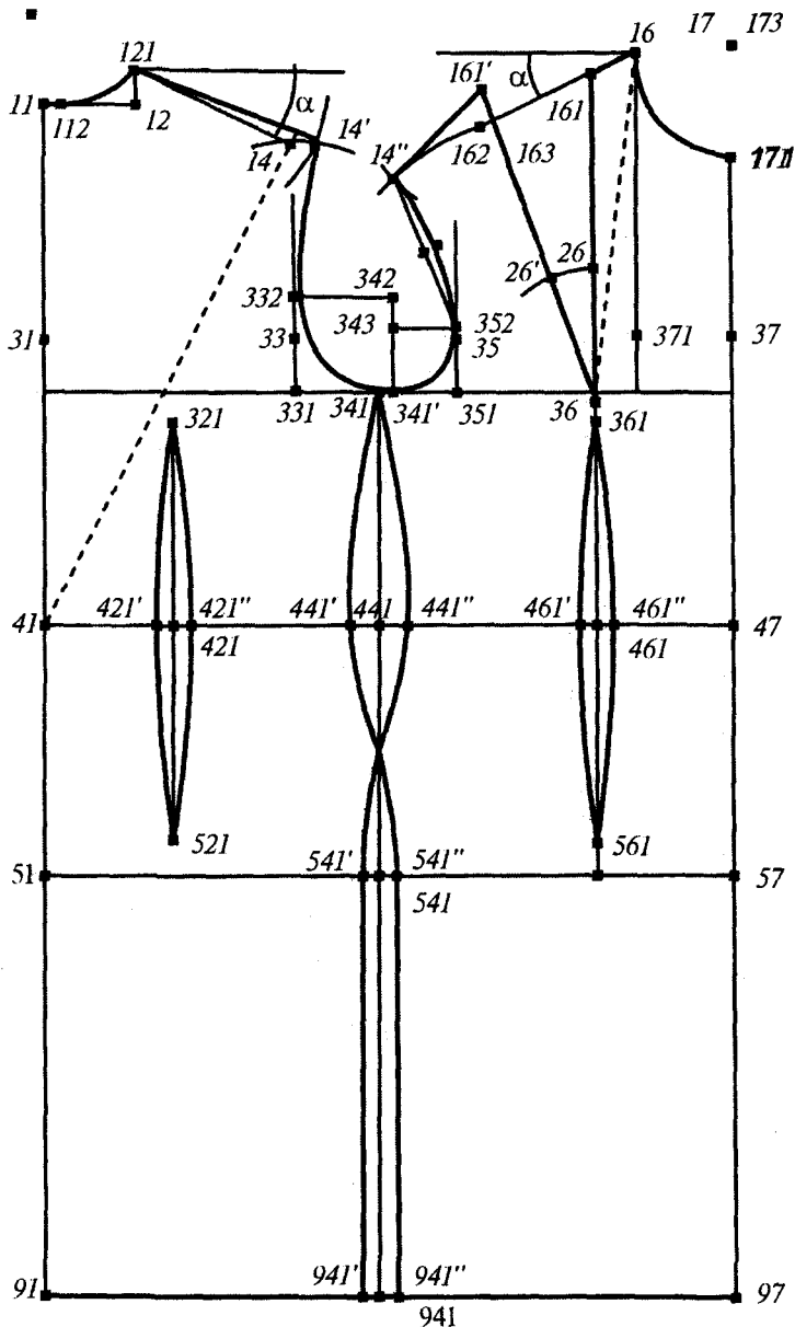
I.4.3.1-rasm. Trikotaj polotnodan ayollar yelkali buyumi asosiy konstruksiyasi.
