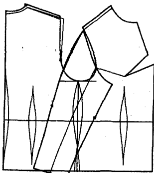
3.33-rasm (a, b). Yaxlit bichilgan yengli va qirqma yon bo'lakli konstruksiyani qurish.
