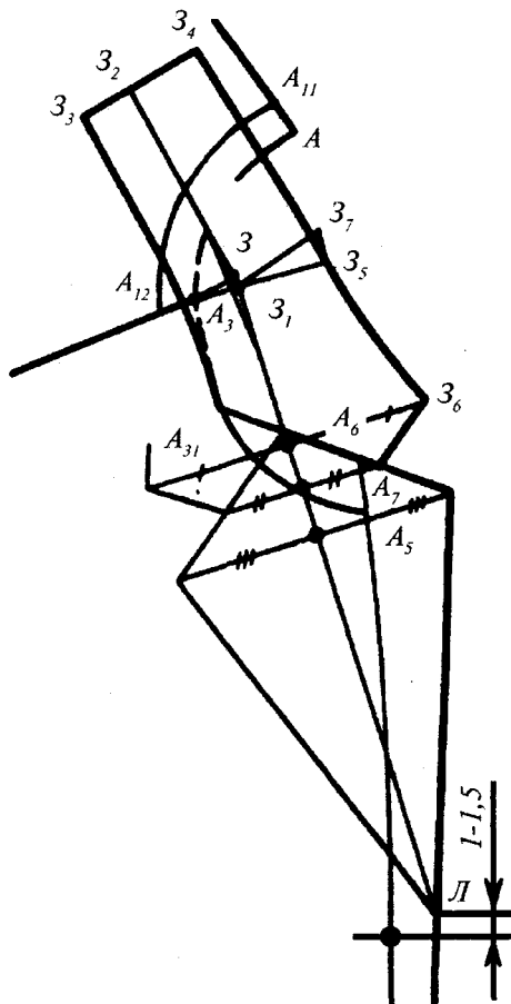
2.45-rasm. Pidjakkbop yoqaning chizmasi.
