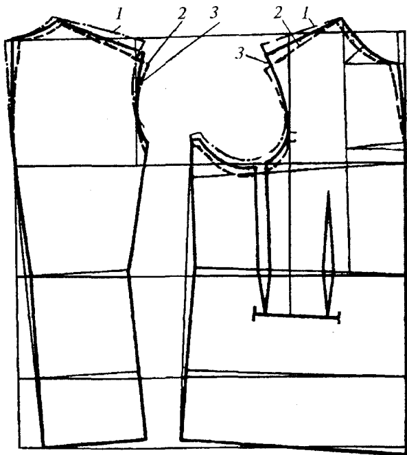
2.73-rasm. Ayollar paltosining konstruksiyasi: normal yelkali (uzluksiz chiziq), past yelkali (punktir chiziq) va baland yelkali (shtrix—punktir chiziq) qomatlariga mo'ljallangan.
