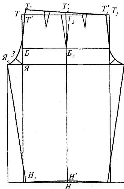
3.43-rasm. Ayollar lozimining konstruksiyasi.
