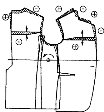
5.14-rasm. Uzun orqa bo'lak.
