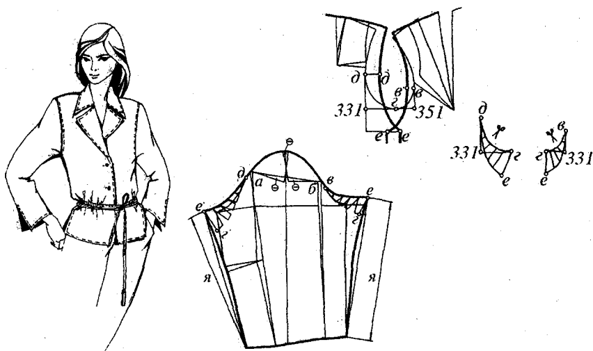
3.22-rasm. Yelka yostiqli, yelka choki uzaytirilgan va chuqurlashtirilgan o‘mizli buyumning bir chokli o‘tqazma yengini modellashtirish sxemasi.
