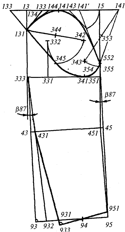
2.34-rasm. Nim yopishgan siluetti palto yengining bazaviy konstruksiyasi.
