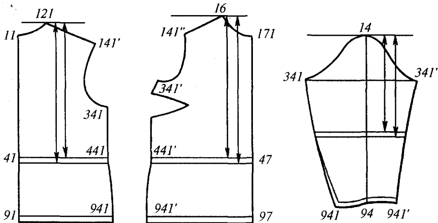
2.63-rasm. Trikotaj polotning kirishuvchanligi hisobga olingan holda andazalarning o'lchamlari o'zgarishi.
