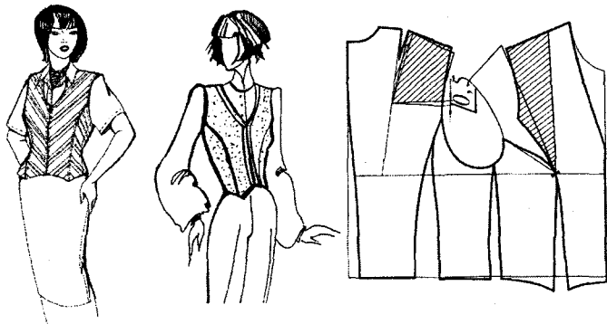
3.5-rasm. O‘miz chizig‘idan va bo‘rtma markazlaridan o‘tgan chok.
