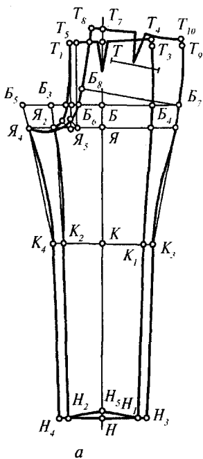
2.47-rasm. Erkaklar shimining konstruksiyasi: a — ЦНИИШП uslubi bo'yicha; b — ЕМКО.
