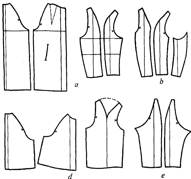
1.23-rasm. Reglan bichimli kiyimning asosiy detallari.
