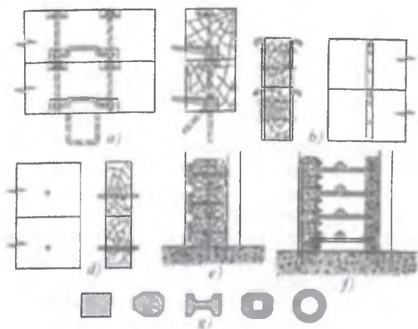
6.7-rasm. Shandor sxemalari: a,b,d yog'och; e,f metall; g temir-beton
