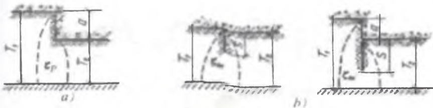
3.19-rasm. Pog'ona va ichki shpunt fragmentlari sxemalari.
