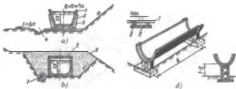
5.50-rasm. Temir-betonli novlar: a–trapetsiya shaklidagi yig‘ma (1,2,3- yig‘ma bloklar, 4–suvni olib ketuvchi ariq); b–yopiq monolitli (1–drenaj; 2–temir-betonli plita; 3–qayta ko‘mish); d- ko‘ndalang kesimi egri chiziqli yig‘ma (1 -nov seksiyasi; 2 tayanch; 3 suv o‘tkazmaydigan zichlagich).
