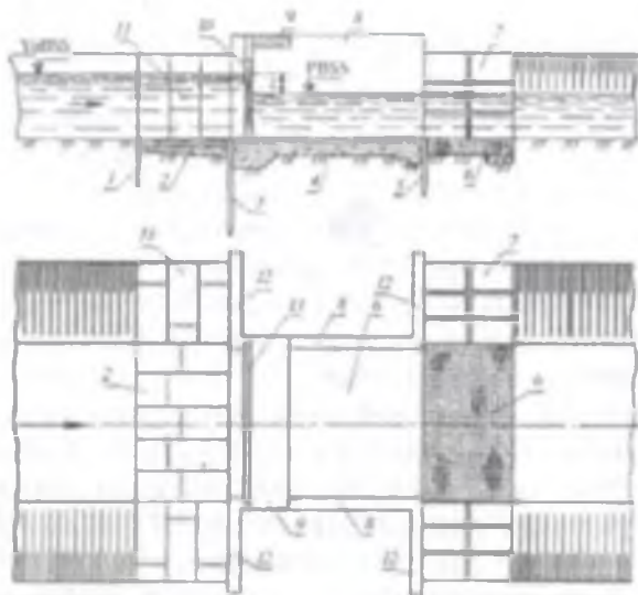
5.5-rasm. Ochiq rostlovchi inshoot: 1–ponur oldidagi shpunt; 2–ponur; 3–markaziy shpunt; 4–suv urilma; 5 pastki shpunt; 6–risberma; 7- pastki byef qiyaliklarini plitalar bilan mustahkamlash; 8–yon devorlar; 9 xizmat ko‘prigi; 10–zatvor; 11 –yuqori byef qiyaliklarini plitalar bilan mustahkamlash; 12 teskari filtr.
