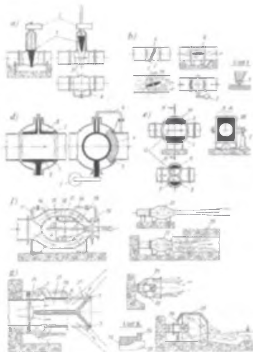
6.34-rasm. Suv bosimini zavvor joylashgan korpus orqali inshootga uzatuvchi chuqur joylashgan zavvorlar: a yassi zadviykalar; b-diskli; d-sharsimon; e-buriluvchi silindrlilik; f-ignasimon; g-konusli; 1-zadviykaning yopuvchi ponasimon disk; 2-zavvorlar va zadviykalar uzatmalari; 3 zavvorni zichlash elementlari (bronzali yoki rezinali); 4 baypas; 5,6-mos ravishda diskning yopilgan va ochilgan holatlari; 7 diskning suyiriligi va momentning paydo bo'lishi; 8-sharsimon zavvor qisqa quvuri; 9 segmentli sirtli zichlagich; 10,11 mos ravishda bir valli va ikki valli zavvor vallari; 12-vallarning yopilgan holati; 13-A bo'shliqni oзуqalantiruvchi quvur; 14-ignasimon zavvor korpusi; 15-ignasimon zavvorni ko'taruvchi qirra; 16-qo'zg'almas kapsula; 17-ishchi ignali qo'zg'aluvchi plunjer; 18-B bo'shliqdan suv chiqaruvchi quvur; 19-igna cheti orqali A bo'shliqdagi suv chiqaruvchi mexanik klapan; 20-havo keltiruvchi kollektor; 21,22-mos ravishda atmosferaga va yopiq quvurga suv chiqaruvchi ignasimon zavvor qurilmasi; 23-shikastlanmaydigan quvur devorli kavitatsiya viloyati; 24-konusli zavvor qo'zg'almaydigan patrubkasi; 25-konus 27 ni ko'taruvchi qirra; 26-harakatlanuvchi patrubka; 28-konusli zavvorga o'rnatilgan nasadka; 29-oqimga havo keltiruvchi tirqish; 30-inshootga o'rnatilgan so'ndiruvchi kamera.
