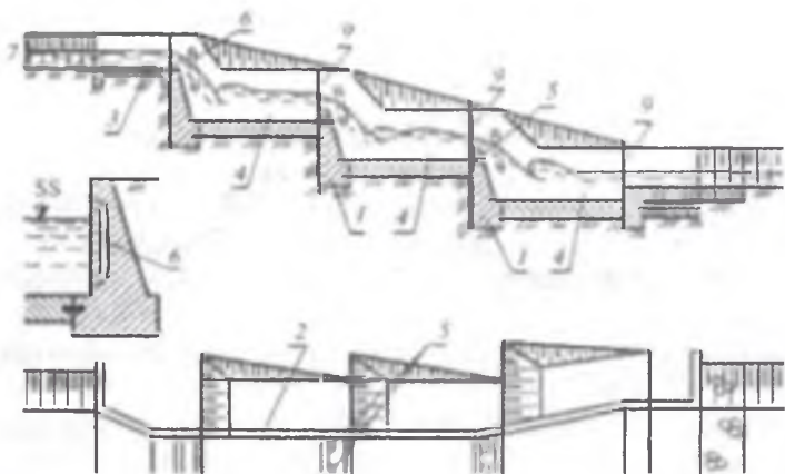
5.26-rasm. Ko'p pog'onali sharshara: 1-tushish devori; 2-yon devorlar; 3-ponur; 4-suv urilma quduq; 5-suv tushadigan tirqish; 6 havo quvurlari; 7-keluvchi kanal; 8-ketuvchi kanal; 9- deformatsiya choklari.
