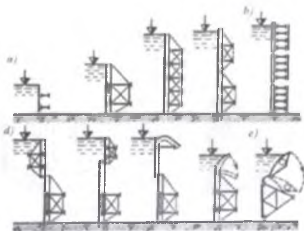
6.10-rasm. Asosiy yassi zatvor turlarining sxemalari: a-yakka holdagi; b-seksiyali; d-ikki qatorli; e-klapanli.
