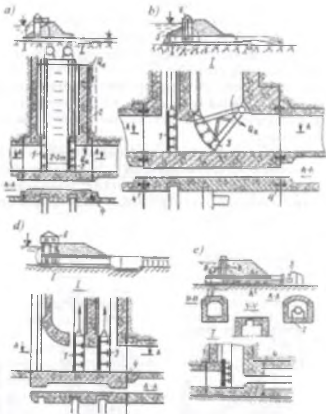
6.43-rasm. Gruntli to'g'onlardagi quvurli suv tashlagichlar mexanik jihozlari: a, b—to'g'ondagi minora bilan; d kirishdagi minora bilan; e—quvurdagi asosiy zatvor bilan; 1- avariya-ta'mirlash zatvorlari; 2 havo yuboruvchi quvur; 3—asosiy zatvor; 4 choklar zichlagichlar bilan; 5 ta'mirlash zatvori; 6—xodimlar binosi; 7—galereya quvurlar bilan.
