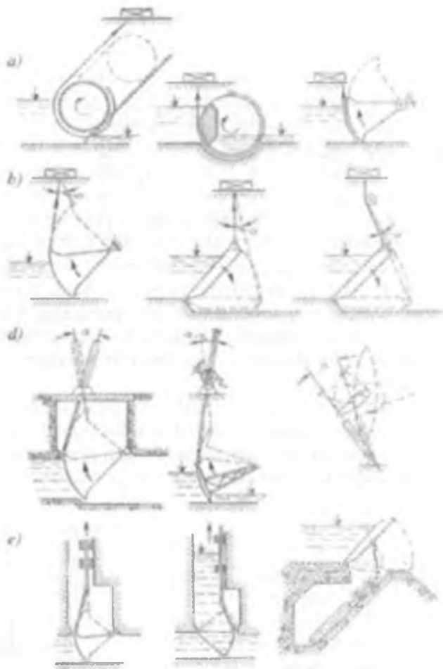
6.39-rasm. Aylanuvchi zatvorlarni mexanizmlarga ulash sxemalari: a -egiluvchan o'raladigan tortqichli; b o'zgaruvchan burchakli egiluvchan tortqichli; d tebranuvchi uzatmali; e krivoship-shatun uzatmali.
