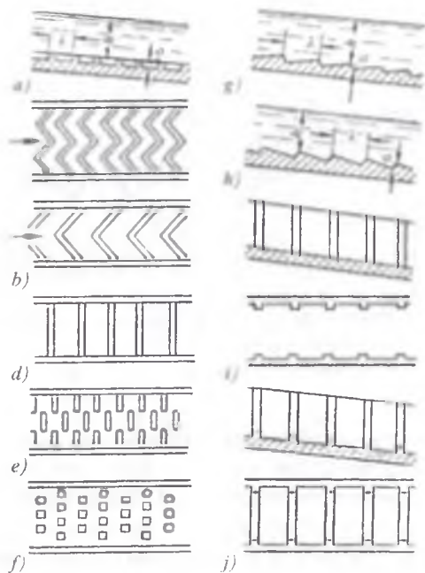
5.35-rasm. G'adir-budurliklar turlari:
