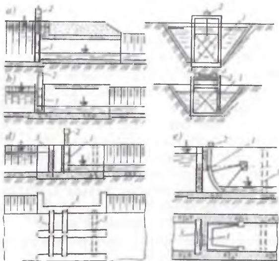
6.41-rasm. Rostlagichlarning mexanik jihozlari:
