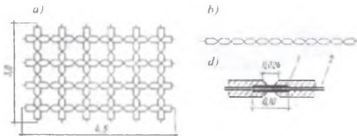
7.24-rasm. Egiluvchan temir-betonli panjaralar:
