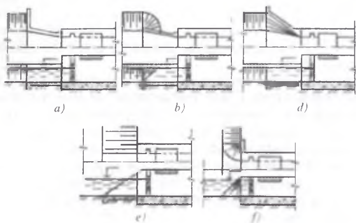
5.6-rasm. Kanal bilan inshoot kirish qismini birlashtiruvchi devor turlari: a–kengayib boruvchi teskari devor; b sho‘ng‘uvchi devor; d–egri devor; f–konusli teskari devor.
