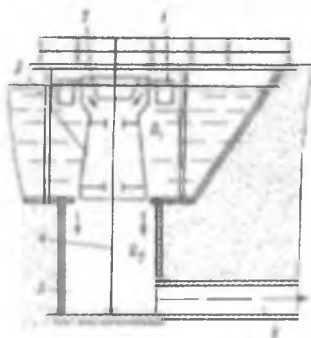
6.49-rasm. Suv bilan o‘zaro ta‘sir etuvchi zatvor-avtomat sxemasi: 1 po‘kak; 2-trapetsidal vodoslivli voronka; 3–avtorostlagich korpusi; 4–yo‘naltiruvchi o‘q; 5–quduq; 6–quvur.
