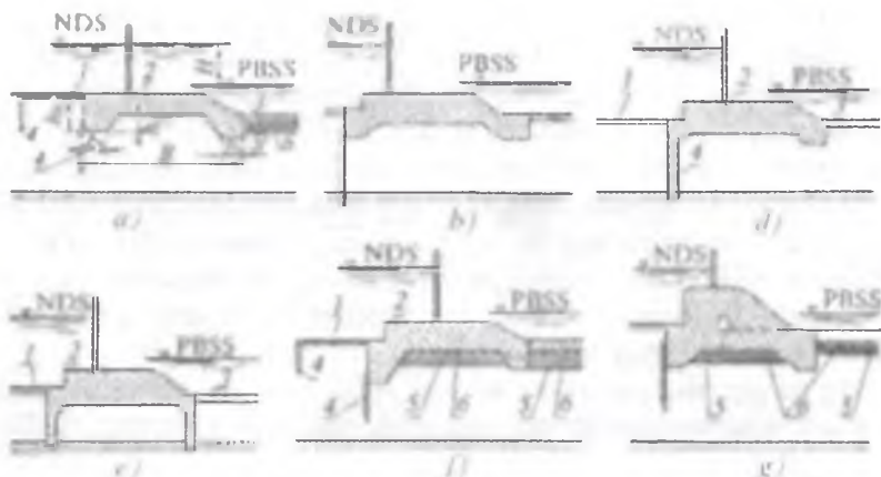
3.25-rasm. To'g'onning suv o'tkazmaydigan qismining yer osti konturi sxemalari: a,b, d, e, drenajsiz; f, g - gorizontaal drenajli; 1 – ponur; 2 – suv urilma; 3 – risberma; 4 – shpunt; 5 – teskari filtr; 6 – drenaj.
