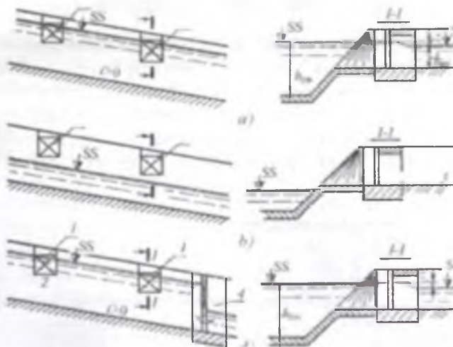
5.18- rasm. Dimlovchi inshoot o'rnatilganda kanalning ishlash rejimi: a- dimlovchi inshoot bo'lmaganda kanalning normal ishlashi; b- kanaldan minimal suv sarfi o'tkazilganda; d- dimlovchi inshoot o'rnatilganda suv sathining dimlanishi; 1- suv oluvchi rostlagich; 2- katta kanal; 3- kichik kanal; 4- dimlovchi inshoot.
