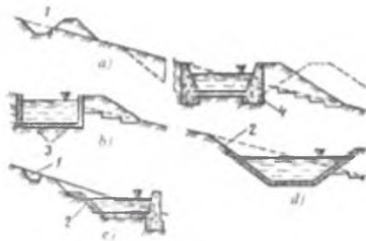
5.49-rasm. Tog' yon bag'irlaridagi novlar: a - monolit; b - yig'ma blokli; d - qoplamali; e - birikmali kesim; 1 - tog'da joylashgan kanal; 2 - plitalar bilan mustahkamlash; 3 - Γ-shaklidagi bloklar; 4 - tirkak devor.
