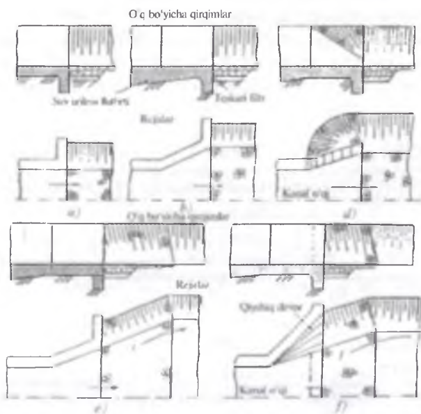
5.10-rasm. Oʻrta qism bilan ketuvchi kanalni birlashtiruvchi devor turlari: a—teskari devor; b kengayuvchi teskari devor; d shoʻngʻuvchi devor; e teskari devor; f—egri devor.
