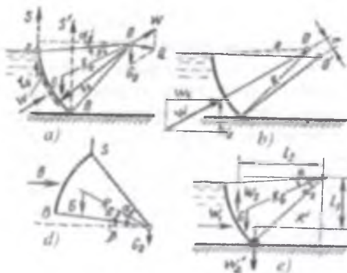
6.25-rasm. Segmentli zatvor ko'tarib - tushirish kuchlari va ustuvorlik hisobi sxemasi.
