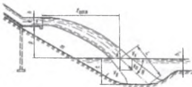
5.40-rasm. Konsolli sharshara gidravlik hisobi sxemasi.
