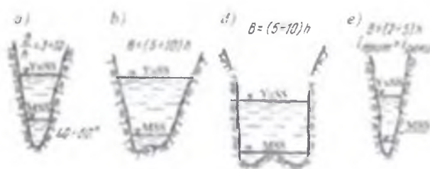
7.3-rasm. Daryoning yuqori togʻli uchastkalaridagi koʻndalang kesimlari: a–uchburchakli; b–trapetsiyali; d–toʻgʻri burchakli; e–quyilishi.
