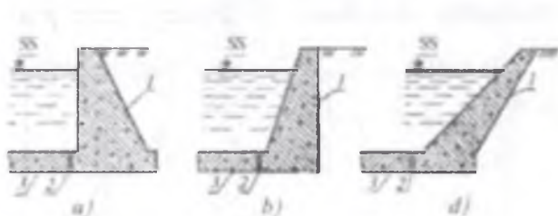
5.8- rasm. Massiv betonli yon devor turlari:
