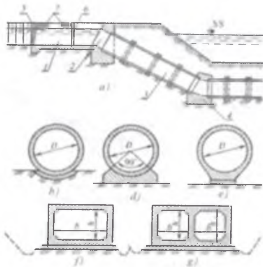
5.42-rasm. Kanal tagidan o'tkazilgan dyuker konstruksiyasi: a -bo'ylama qirqim; b,d,e -doiraviy quvurlar; f,g -mos ravishda bir va ko'p ko'zli quvurlar; 1 kirish qismi; 2 kirish kallagi; 3-bosimli quvur; 4-ankerli tayanch; 5-panjara; 6-zatvor; 7 -xizmat ko'p rigi.
