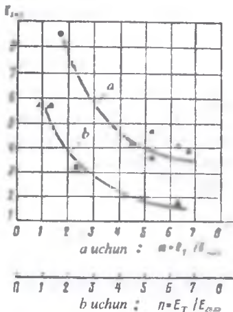
4.7-rasm. Umumlashtirilgan zaxira koeffitsiyenti qiymatining zamin xususiyatlariga bog'liqlik grafigi: a, b - massiv-kontrfors ( h_1=116 m) va arkali ( h_1=100 m, keng storvli ( L/h_1=4 ) to'g'on; L-to'g'on uzunligi; h_1 - to'g'on balandligi.
