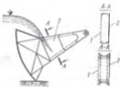
6.22-rasm. Ustidan suv quyiladigan yassi oyoqli zatvor.
