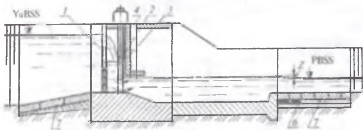
5.17-rasm. Diafragmali rostlagich: 1 - ta'mirlash zatvori (shandor); 2 - asosiy zatvor; 3 - diafragma; 4 - shandorlar taxlab quyiladigan paz; 5 - risberma; 6 - risberma plitalari tagidagi teskari filtr; 7 - betonli plita.
