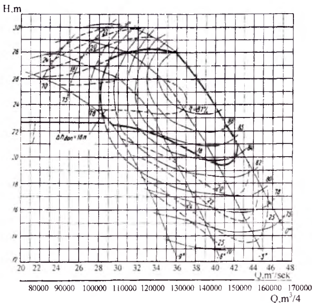
3.7-rasm. OPV10 – 260 vertikal o‘qiy nasos universal xarakteristikasi ( \Delta h_{rux} – kavitatsiya zaxirasi chizig‘i)
