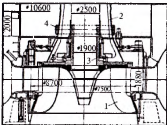
1.1-rasm. Krasnoyarsk GESi gidroturbinasi:
