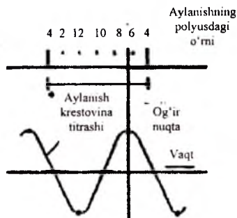
1.10-rasm. Ossillogramma bo'yicha generator rotoridagi mavozanatlilik yukining mahkamlanishi joylarini aniqlash. Aylanishlar belgi datchigi va titrash datchiklari bir vertikal tekislikda o'rnatilgan
