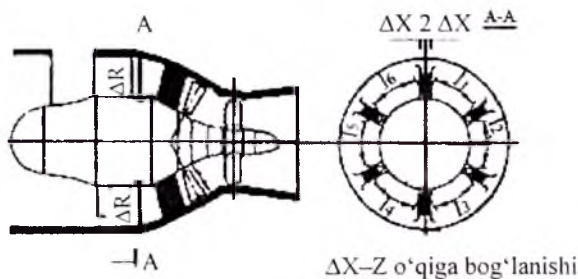
1.8-rasm. Kapsulali agregat oquvchi qismidagi nazorat oʻlchovlari
