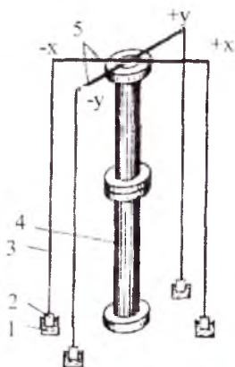
4.16-rasm. Torlar bo'yicha markazlanganda o'qlarni belgilash va torlarni osish sxemasi: 1-moyli chelak; 2-yuk; 3-tor; 4-val; 5-tallar osish chambaragi.
