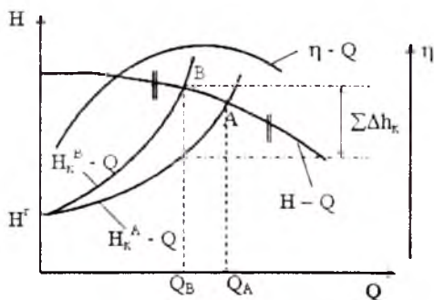
3.8-rasm. Nasosning ish rejimini drossellash usuli bilan roslash grafigi
