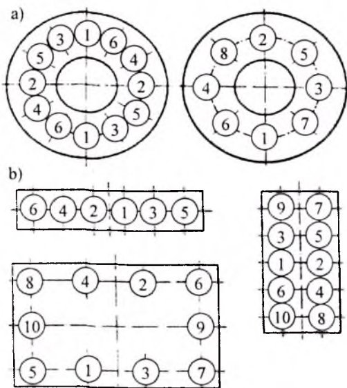
4.1-rasm. Rezkali birikmalarni tortish ketma-ketligi, a-flanetsli; b-tasmali va to'g'ri to'rtburchakli.
