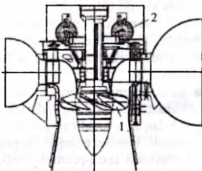
1.2-rasm. Vilyuysk GESi gidroturbinasi:
