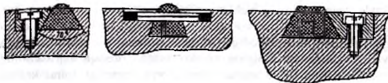
1.4-rasm. Yo‘naltiruvchi apparat kurakchalari zichlamalari
