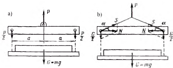
4.9-rasm. Egilishga (a) va siqilishga (b) ishqalaydigan traverslarning hisobiy sxemalari, egilishga ishlaydigan travers hisobi.
