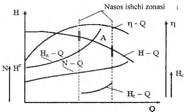
3.5-rasm. Markazdan qochma nasosning ishchi xarakteristikasi
