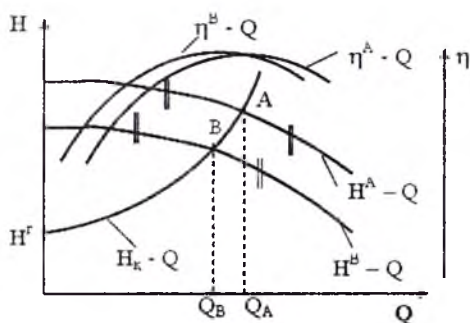
3.9-rasm. Nasosning ish rejimini nasos vali aylanishlar sonini o'zgartirish usuli bilan rostdash grafigi
