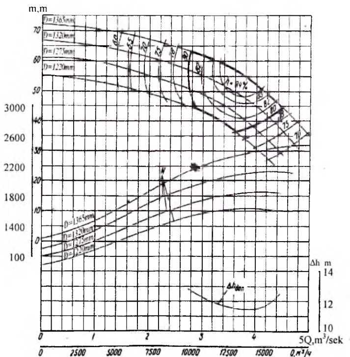
3.6 – rasm. Vertikal markazdan qochma 1000V – 4/53 markali nasosning universal xarakteristikasi ( \Delta h_{rux} – kavitatsiya zaxirasi chizig'i)
