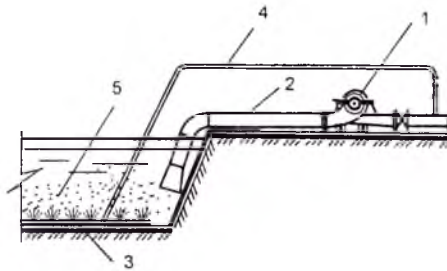
3.16-rasm. Avankamerani loyqa bosishini oldini olish qurilmasiga ega boʻlgan suv qabul qilish inshootining yangi konstruksiyasi
