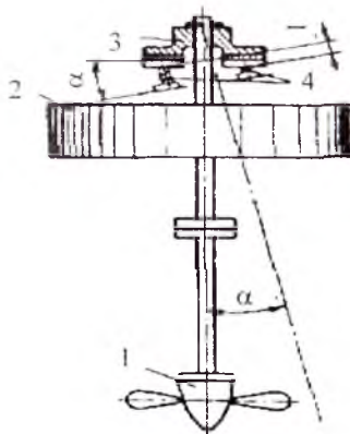
4.15-rasm. Podpyatnik segmentlarining noto'g'ri o'rnatilishi bilan yuzaga keladigin agregat vali chizig'ining qiyalig:
