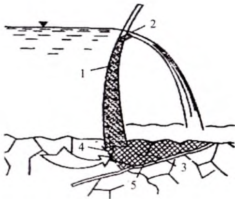
2.1-rasm. Mal'passe (Fransiya) to'g'onining avariya holati:
