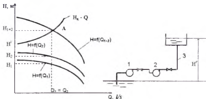
3.11-rasm. Nasoslarning ketma – ket ishlashi grafigi va sxemasi:
