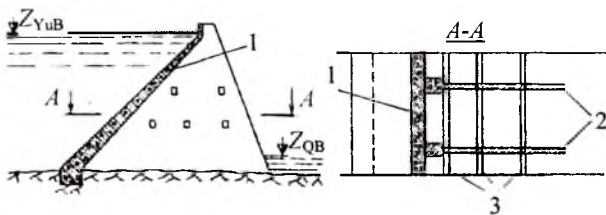
2.7-rasm. Kontrfors to'g'on: 1 – temir – beton plitalar; 2 – kontrforslar; 3 – mahkamlash balkalari
