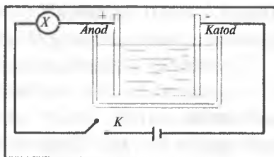
1-rasm. Elektrolitlarning elektr o'tkazishiga oid elektr zanjiri.
