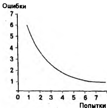
Рис. 1. Отрицательное ускорение
