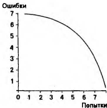
Рис. 2. Положительное ускорение
