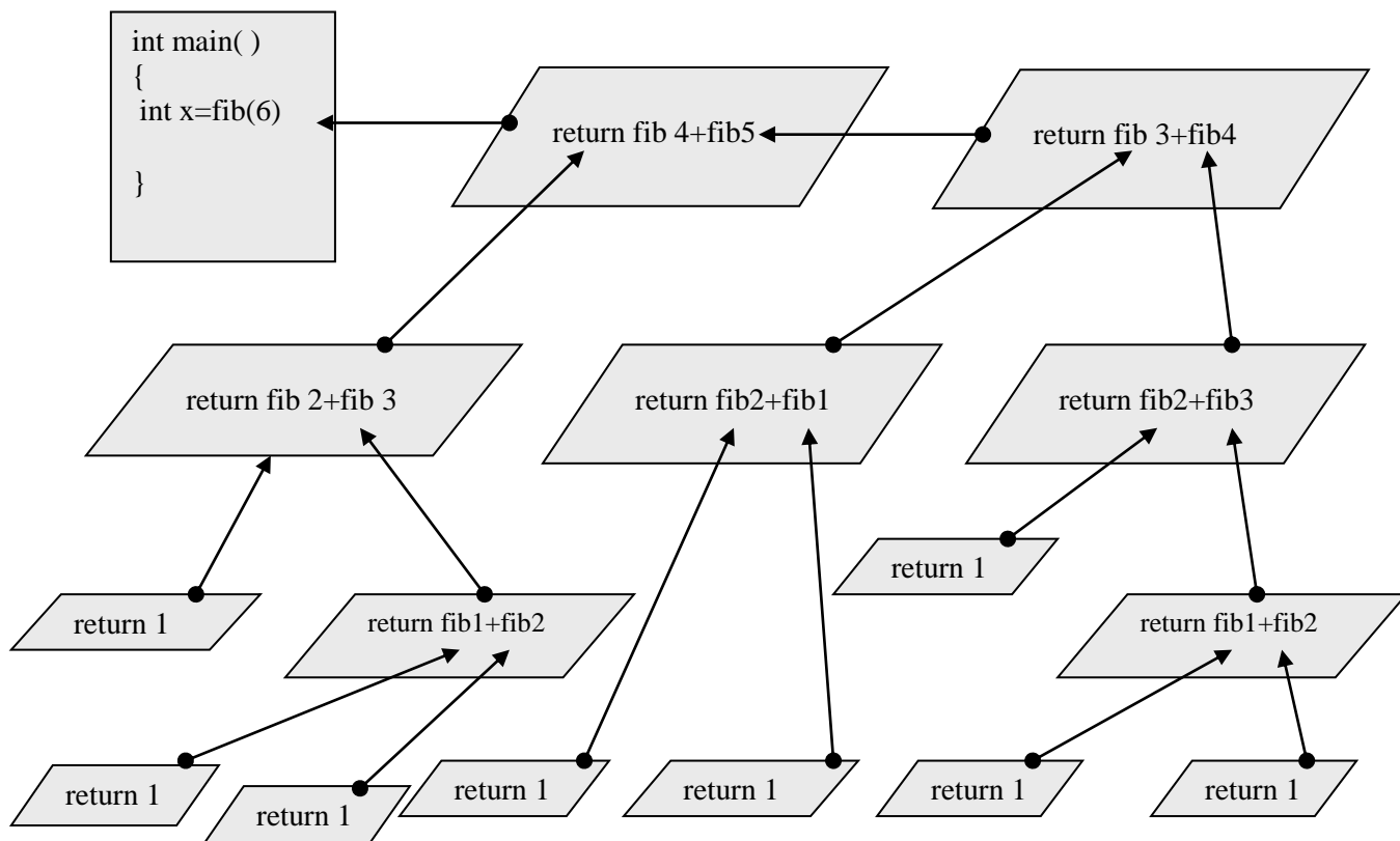
5.5. – расм. Рекурсив функцияларнинг қиймат қайтариши.
