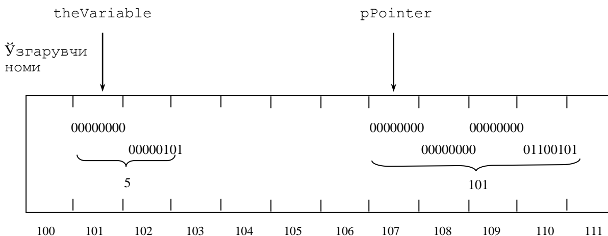
8.3. – расм. Хотирани тақсимланиш схемаси
