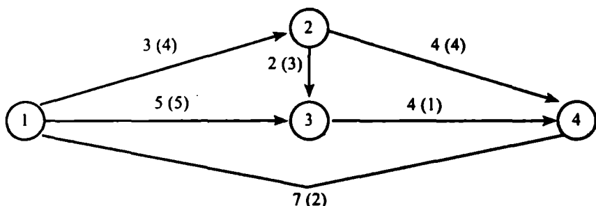
4.2-rasm. Texnologik jarayonning to'rsimon grafi.
