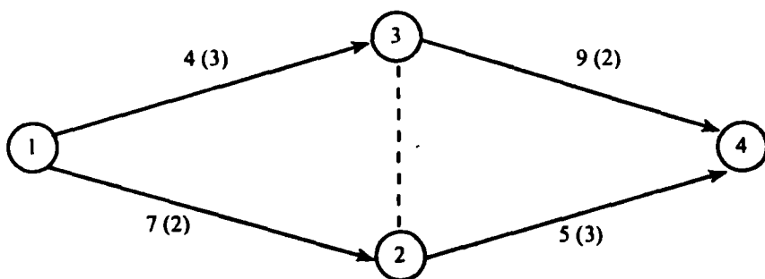
4.1-rasm. To‘rsimon grafiga misol
