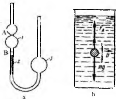
3.3-rasm. Yopishqoqlik koeffitsiyentini aniqlashning viskozimetriya (a) va Stoks (b) usullari. 1,3-o'lchov hajmlari, 2-kapillyar, F_A -Arximed kuchi, mg -ogirlik kuchi, v -tezlik
