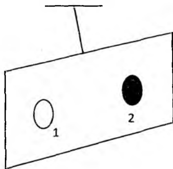
8.19-rasm. Yorug'lik bosimini o'lchashdagi Lebedev tajribasi qurilmasi. 1- ko'zgusimon sirt, 2- qoraytirilgan sirt
