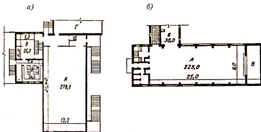
Рис. 11.6.4. Гимнастический зал с комплексом подсобных помещений: а — гимнастический зал с комплексом, б — гимнастический зал, совмещенный с актовым залом
