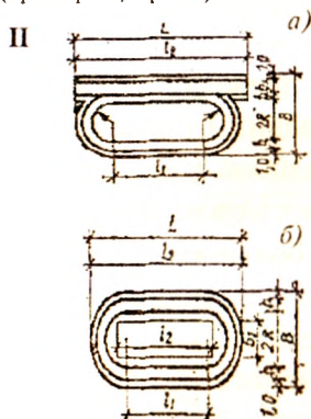
Рис. 12.7.1.4. Примеры организации залов манежей: I — план манежа: 1 — прыжки в длину, 2 — прыжки с шестом в длину, 3 — прыжки в длину, 4 — прыжки с шестом, 5 — замкнутая дорожка 200 м, 6 — прямая дорожка 150 м, 7, 8 — толкание ядра, 9 — участок дорожки с виражом, 10, 11 — места для прыжков в высоту, 12 — метание диска и молота, 13 — метание копья, 14, 15 — места для прыжков в длину и тройного, 16 — сетка, 17 — игровые площадки, 18 — футбольное поле, 19 — скамейки, 20 — помещение для гимнастики, 21 — трибуны; II — габаритные схемы основных залов манежей: а — прямая дорожка примыкает к круговой, б — прямая дорожка расположена в пределах внутреннего контура
