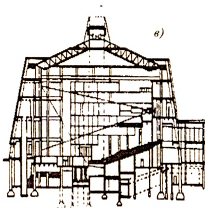
Рис. 14.1.6.1. Конструктивное решение здания киноконцертного зала в г. Душанбе (арх. С. Сутягин): а — общий вид, б — план, в — разрез
