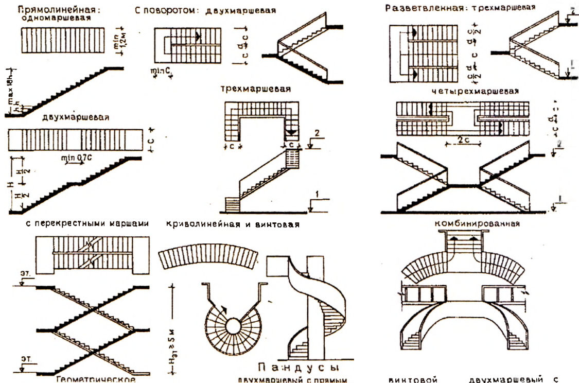
Рис. 9.1.7. Схемы вариантов устройства лестниц в общественных зданиях
