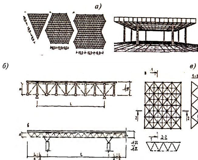
Рис. 5.8. Пространственные перекрестно-стержневые конструкции:
