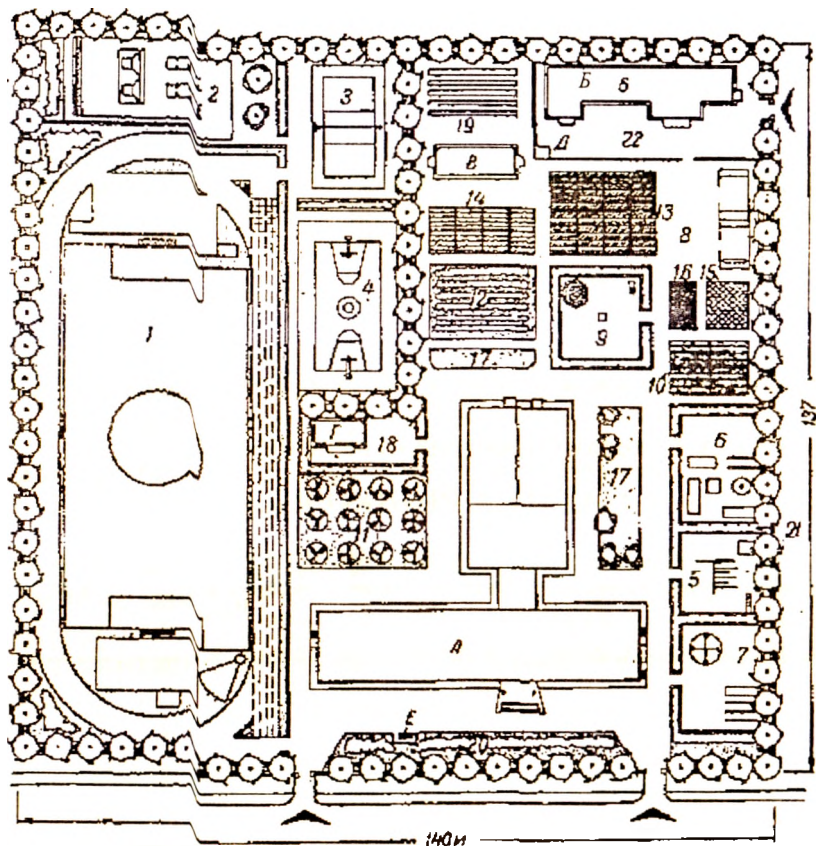
Рис. 11.9.2. Схема генерального плана школьного участка: А — здание, Д — сарай, Е — физкультурный корпус, В — теплица, Г — теневой навес, подвижных игр — флагшток; 1 — спортивное ядро, 2 — площадка для шадка, 5 — гимнастическая площадка, 6 — площадка для детских спортивных развлечений (I–IV кл.), то же (V–IX кл.), 8 — зоологическая площадка, 9 — географическая и метеорологический сад, 12 — участок начальных классов, 11 — плодово-ягодный сад, 13 — участок питомник плодово-ягодных и декоративных растений, участок сеянцев овощных культур, 14 — участок полевых культур, 15 — тивных растений, 16 — коллекционный участок, 17 — участок декоративных растений и цветов, 18 — площадка занятий на воздухе, 19 — газоны и декоративная зелень, 21 — ветрозащитная зеленая полоса, 22 — хозяйственный двор
