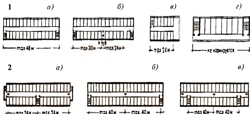
Рис. 9.1.5. Схемы организации коммуникационных связей.
