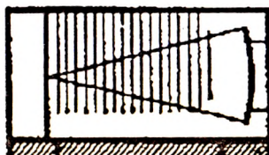
Рис. 14.1.5.6. Схема размещения зрительских мест в залах кинотеатров: а — с двухсторонней эвакуацией, б — с односторонней эвакуацией
