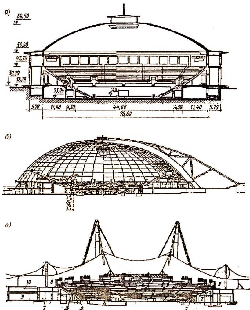
Рис. 12.7.4.3. Примеры большепролетных покрытий: а - Дворец спорта в Тбилиси, купол - сборные железобетонные элементы, б - крытый стадион в Питсбурге (США), купол - монолитный железобетон (пролет свыше 100 м), в - крытый плавательный бассейн в Мюнхене (пролет свыше 100 м)
