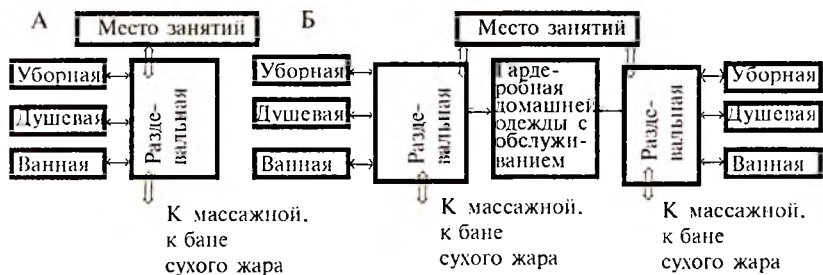
Рис. 12.7.3.2. Функциональная организация взаимосвязи раздевальни с другими помещениями: а — раздевальня для команд по спортивным играм с хранением одежды на крючках, б — то же, с хранением одежды в гардеробе с обслуживанием
