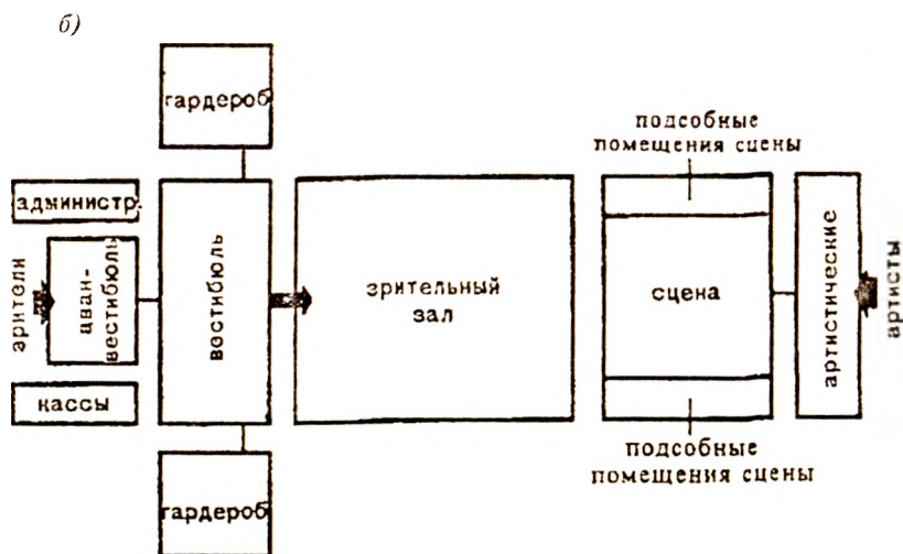
Рис. 9.1.1. Схемы взаимосвязей помещений в общественных зданиях: а — в спортивном зале, б — в театре
