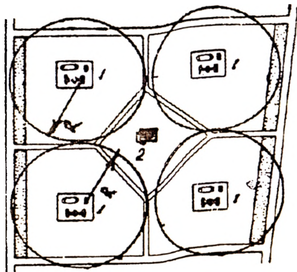
Рис. 11.2.1. Схема организации школьной сети в городских микрорайонах: 1 — школы, 2 — общественные центры микрорайонов, R — радиус обслуживания школы = 750 м
