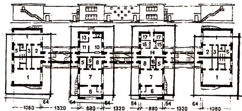
Рис. 4.4. Функциональное зонирование основных и вспомогательных помещений детского сада-яслей: 1, 4 — зоны ясельных групп; 2, 3 — зоны садовских групп и административно-вспомогательных помещений
