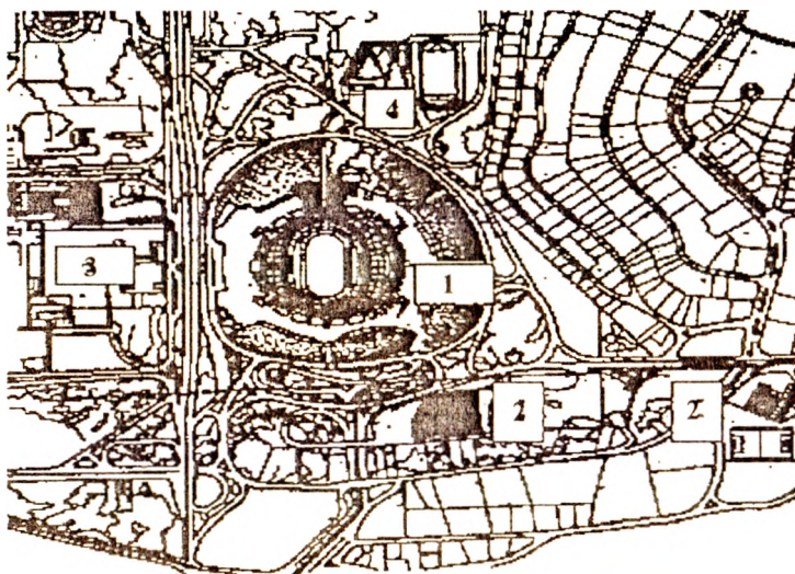
Рис. 12.3.2. Функциональная организация территории стадионов: а – стадион в Лужниках (Москва), б – стадион в Мехико (Бразилия): 1 – центральная арена, 2 – универсальные залы, 3 – бассейн, 4 – малая арена
