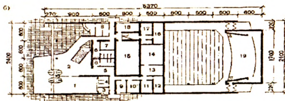
Рис. 14.1.4.2. Приемы планировочных решений однозальных кинотеатров:
