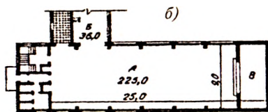
Рис. 11.6.6. Приемы планировочных решений актовых залов: а — стандартный тип актового зала, б — актовый зал, совмещенный с комнатой для музыкальных занятий, в — актовый зал, совмещенный со столовой
