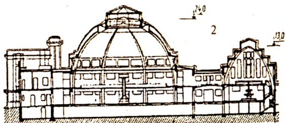
Рис. 15.6.4.3. Пример арочной конструкции с плоскостной кровлей крытых рынков (на примере рынка в Плоешти – Румыния, арх. Т. Соколеску): 1 – интерьер торгового зала, 2 – разрез
