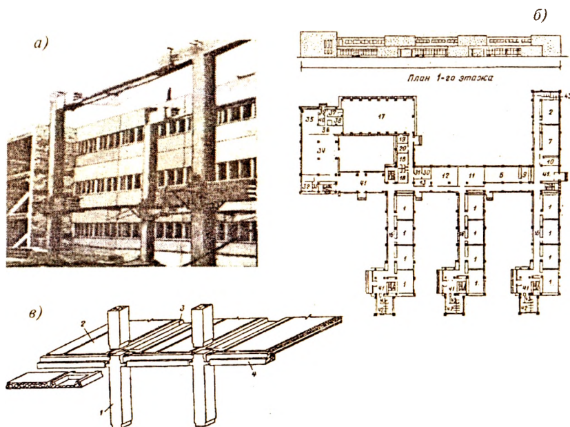
Рис. 11.8.1. Конструктивные системы типовых проектов школ
