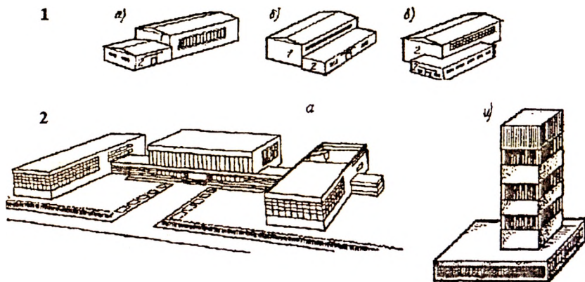
Рис. 12.7.1.1. Примеры композиционных решений одно- и многозальных крытых спортивных корпусов: 1 — однозальные: а — торцовая, б — продольная, в — угловая композиции; 2 — многозальные: а — блочная (арх. Ю. Абрамов и Э. Марьясина), б — многоэтажный спортивный корпус с расположением вспомогательных помещений на первом этаже
