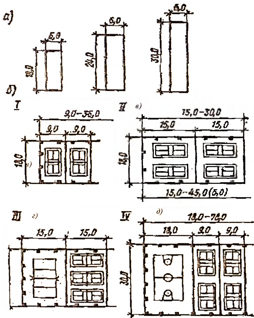
Рис. 12.7.1.2. Примеры компоновки основных залов спортивных сооружений из унифицированных элементов и блоков:
