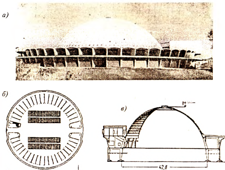
Рис. 15.6.4.7. Пример покрытия рынка куполом из сборных элементов (Сидибель-Аббас, арх. М. Мори): а — общий вид, б — план, в — разрез
