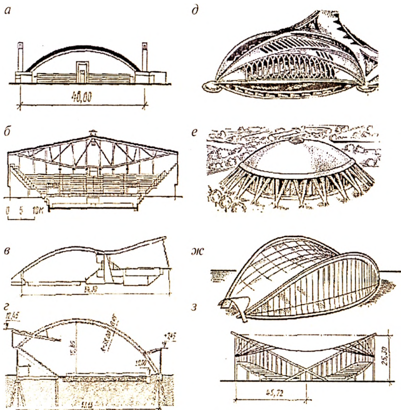
Рис. 12.7.4.1. Примеры конструктивных и архитектурных решений крытых спортивных комплексов: а — спортивный зал в Амстерфорде (Нидерланды), деревянные арки, б — зал с хоккейной ареной в г. Оуду (Финляндия), деревоклассные конструкции, растяжка ферм из круглой стали, в — спортивный комплекс с хоккейной ареной и бассейном в г. Реймсе, деревоклассная балка, г — крытый каток в Гренобле (Франция), деревоклассные конструкции, д — спортивно-зрелищный зал в г. Нордфолде (США), сборно-моноклитный сферический купол, е — крытый велодром Олимпийского комплекса в Монреале (Канада), железобетонные конструкции, ж — крытый стадион с хоккейной ареной в Париже, преднапряженная сетка стальных тросов, з — релей-арена в США, перекрестная сетка тросов
