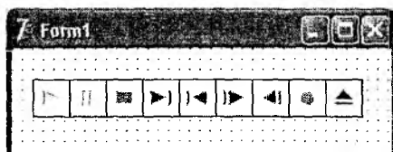
Рис. 9.4. Компонент MediaPlayer.
