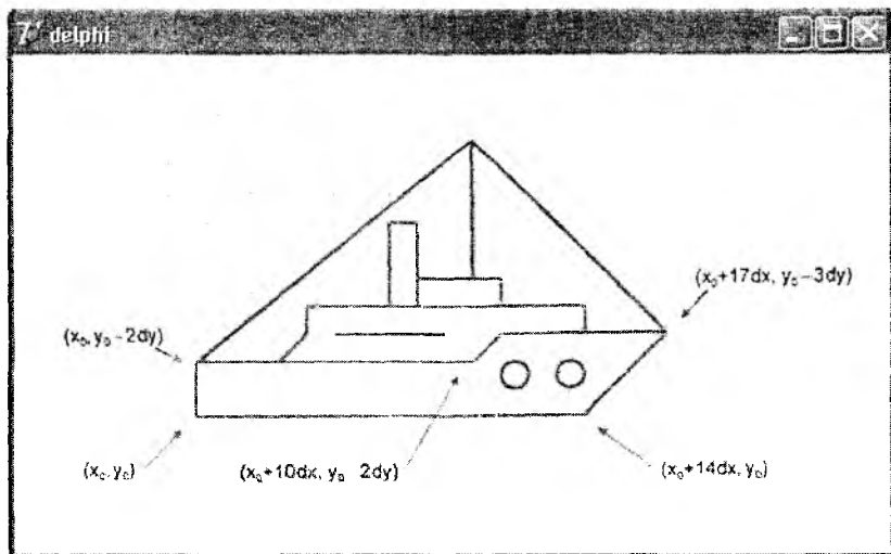
Рис. 9.16. Определение базовой точки изображения.
