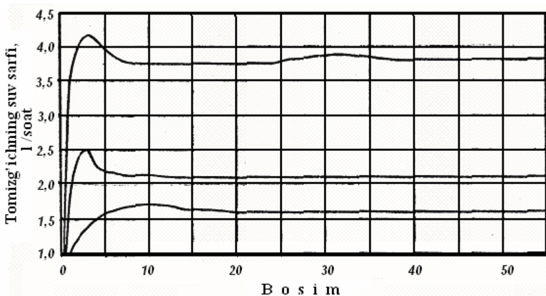
36-rasm. Naan-Tif 20 tomizg'ichining suv sarfi xarakteristikasi
