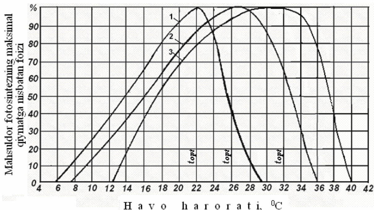
45-rasm. Mahsuldor fotosintezning havo haroratiga bog‘liqligi: 1-bug‘doy; 2-makkajo‘xori; 3-g‘o‘za.
