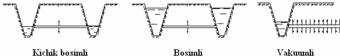
31-rasm. Tuproq ichidan sug'orish tizimining ko'rinishlari
