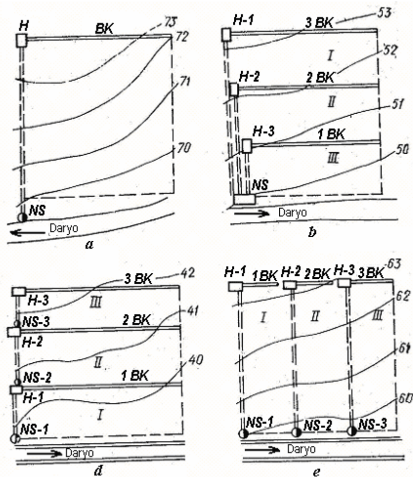
76-rasm. Suv ko‘tarish zonalarini (I, II, III) belgilash, nasos stansiyalari (NS), hovuzlar (H), bosimli quvurlar va bosh kanallarning joylashuvi sxemasi
