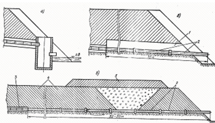
122-rasm. Suv chiqarish inshooti konstruksiyalari: a -quduqli; b -yaxlit qulfakli; d -tishli qulfakli; 1-qulfak; 2-teshiksiz zovur quvuri; 3-qum-shag'alli aralashma; 4-qayta to'kma; 5-kollektor tuproq uyumi
