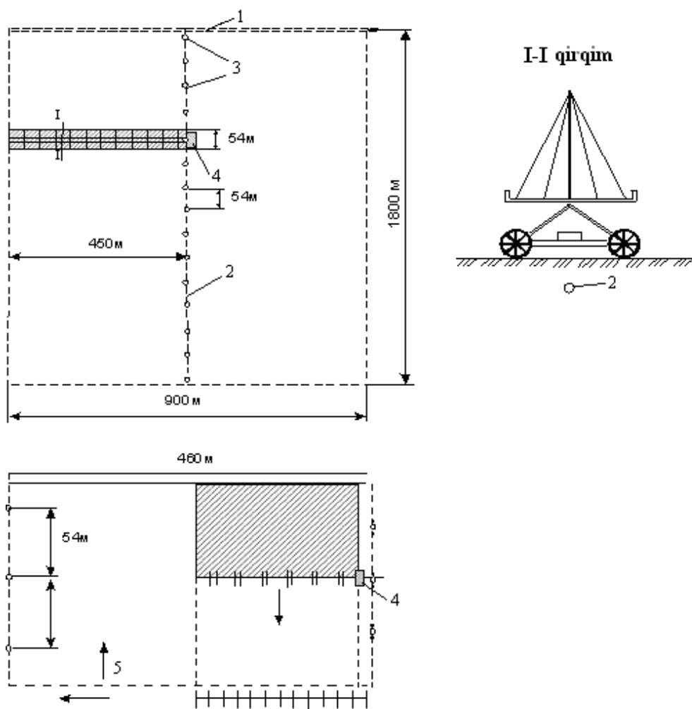
26-rasm. «Dnepr» yomg'irlatib sug'orish mashinasi ishlashining texnologik sxemasi:
