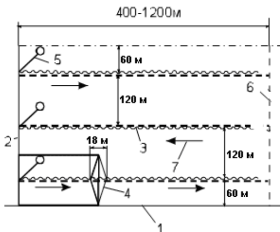
23-rasm. ДДА-100 МА yomg'irli sug'orish agregatining ishlash texnologik sxemasi:
