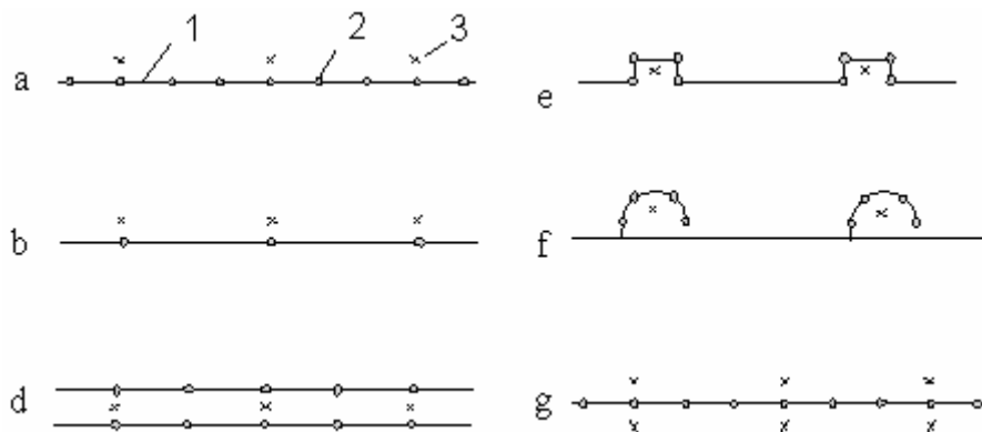
42-rasm. Sug'oruvchi quvurlarning rejada joylashish sxemasi: 1-sug'oruvchi quvur; 2-tomizg'ich; 3-o'simlik; a, b, d, e, f, g-sug'orish quvurlarining o'simlik qatoriga nisbatan joylashish ko'rinishlari
