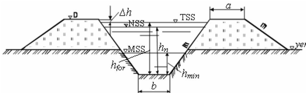
56-rasm. Kanalning koʻndalang kesimi
