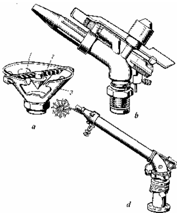
22-rasm. Yomg'irlatish uchliklari: a-urilmali; b, d-purkovchi
