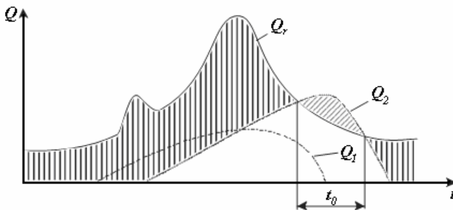
74-rasm. Suv manbasi (daryo) suv rejimining tahlili grafigi
