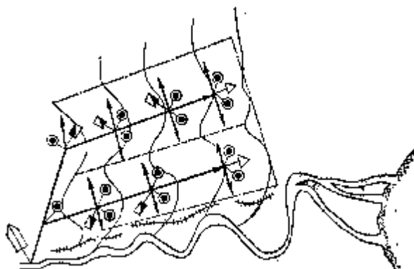
53-rasm. Delta relyefi sharoitidagi sug'orish tarmoqlarining sxemasi
