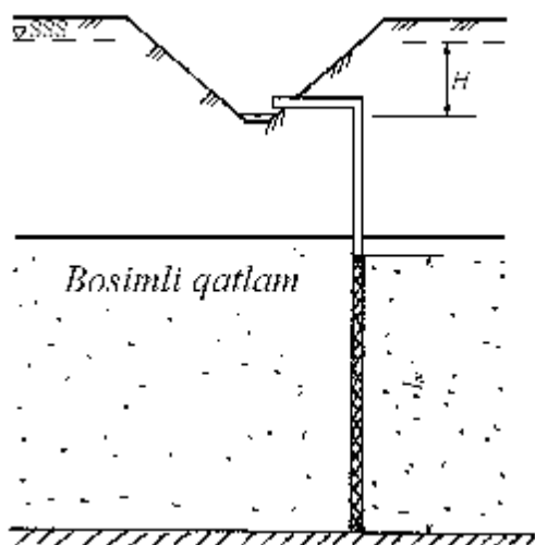
109-rasm. Qurama zovurlar
