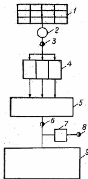
86-rasm. Chorvachilik chiqindi suvlarini sug'orishga tayyorlash sxemasi:
