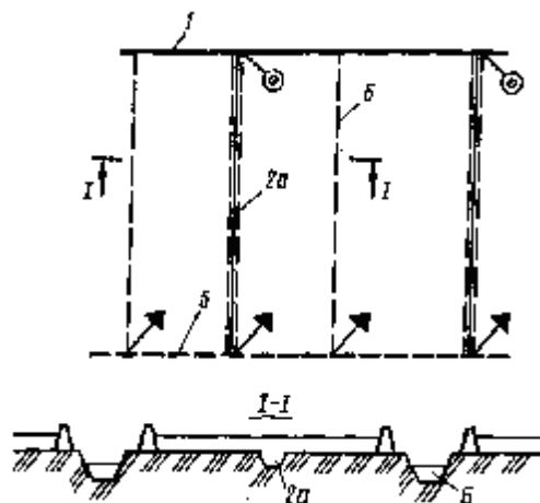
18-rasm. Uzoq Sharq tipidagi sholi kartasi:
