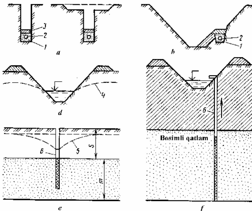
95-rasm. Gidrotexnik ( a,b -yopiq yotiq; d -ochiq yotiq; e -tik; f -qurama) zovur: 1 -qum-shag‘alli filtr; 2 -zovur quvuri; 3 -himoya qatlam; 4, 5 -depressiyalik egrilik chizig‘i; 6 -tik quduq
