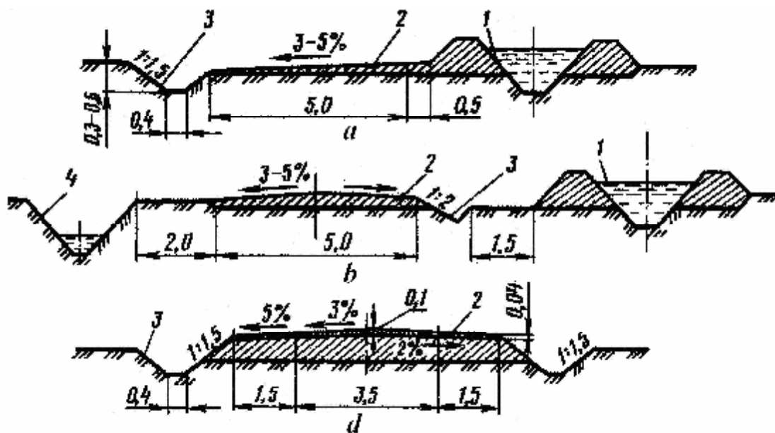
72-rasm. Dala (a, b) va xo‘jalik ichki (d) yo‘l tarmoqlarining ko‘ndalang qirgimlari:
