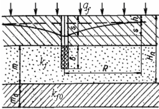
111-rasm. Hosil bo'lgan suv ta'minoti uchun nomukammal tik zovurning hisobiy sxemasi
