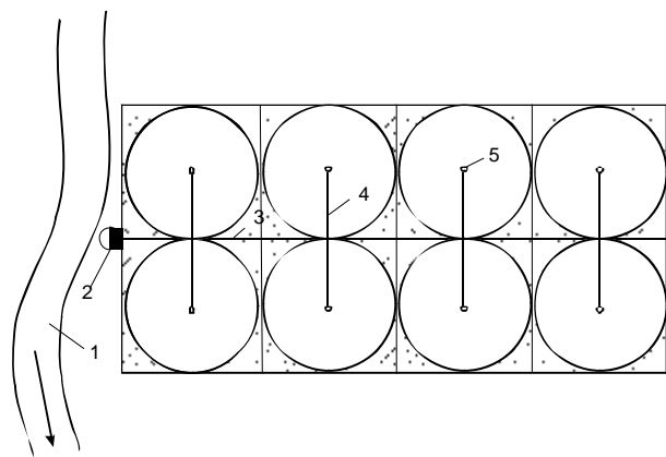
25-rasm. «Fregat» yomg'irlatib sug'orish mashinasi bilan sug'orish sxemasi:
