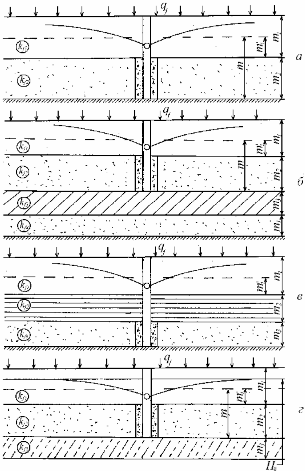
124-расм. Қурама зовурларнинг намунавий филтрацион ҳисобий схемалари:
