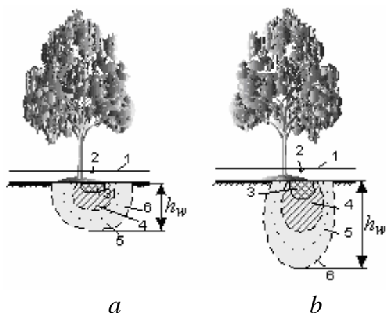
40-rasm. Tomchilatib sug'orishda tuproqning namlanish konturi ( a -og'ir, b -yengil tuproqlarda): 1-sug'oruvchi quvur; 2-tomizg'ich; 3-namlantirish manbai; 4-normal namlangan manba; 5-qisman namlangan joy; 6-namlanish konturi.
