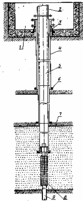
79-rasm. Burg'u qudug'i sxemasi: 1-shaxta; 2-kirish qismi; 3-ustki qism; 4-o'rnatilgan quvur; 5-foydalanish kalonkasi; 6-frezer; 7-suvli qatlam; 8-filtr; 9-tindirgich
