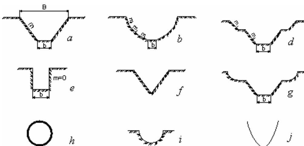
60-rasm. Sug'orish tarmoqlarining ko'ndalang kesimi ko'rinishlari
