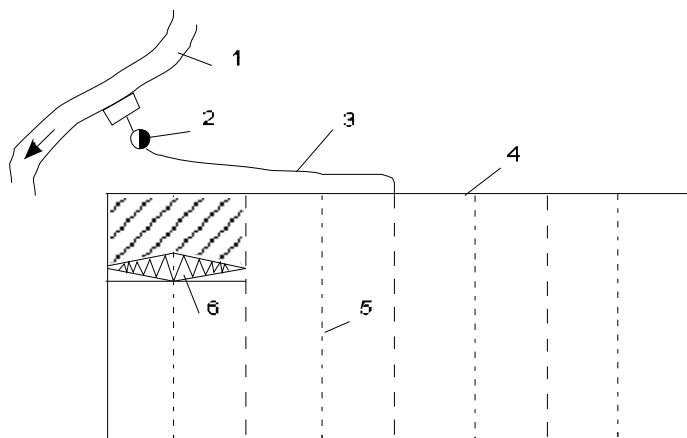
21-rasm. Yomg'irlatib sug'orish tizimi: 1-manba; 2-sun'iy bosim hosil qilish qurilmasi; 3-xo'jalik tarmog'i; 4-shohariq; 5-muvaqqat (suv berish) tarmog'i; 6-yomg'irlatib sug'orish qurilmasi
