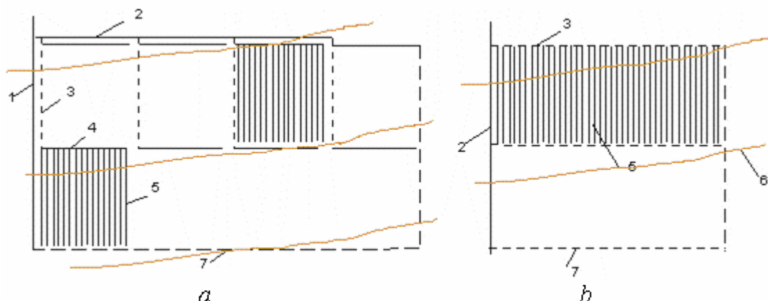
20-rasm. Muvaqqat ariqlarning sug'orish maydonida joylashish (a-bo'ylama, b-ko'ndalang) sxemasi:
