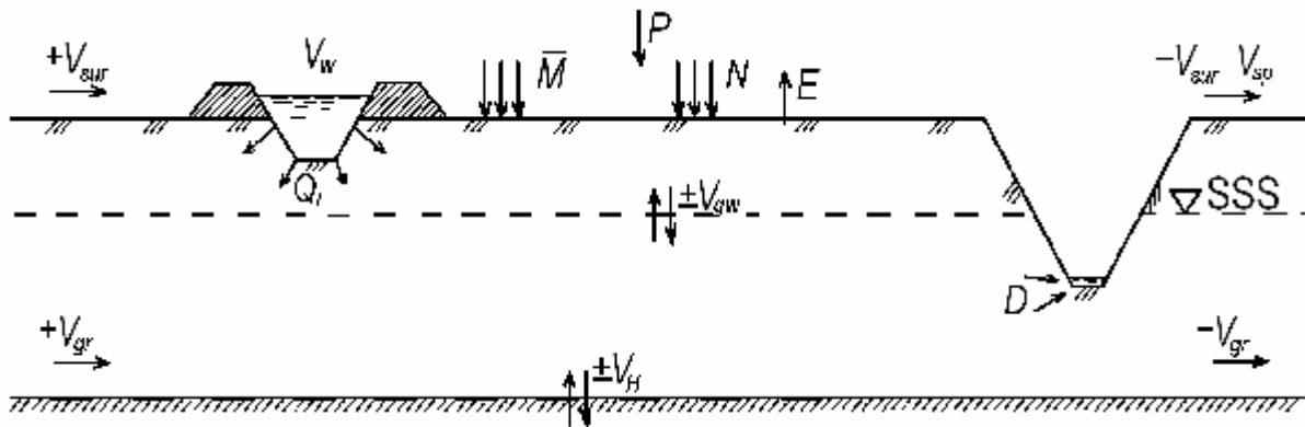
101-rasm. Sug'orish maydonining suv muvozanat sxemasi
