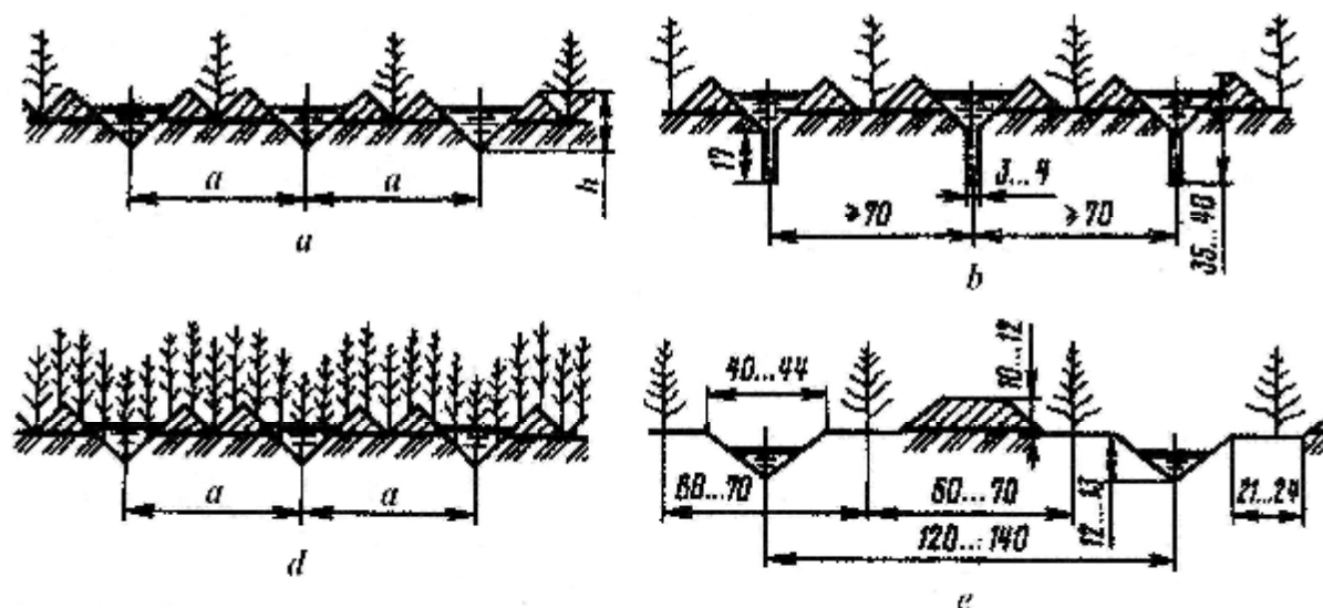
10-rasm. Sug'orish egatlarining konstruksiyalari: a -oddiy, chopiq qilinadigan ekinlar uchun; b -tilma egatlar; d -ekiladigan egatlar; e -supali egatlar (o'lchamlar santimetrd)
