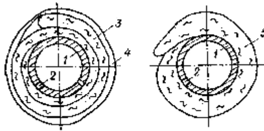
107-rasm. Yotiq zovurlar uchun sun'iy tolali filtrlar konstruksiyasi:
