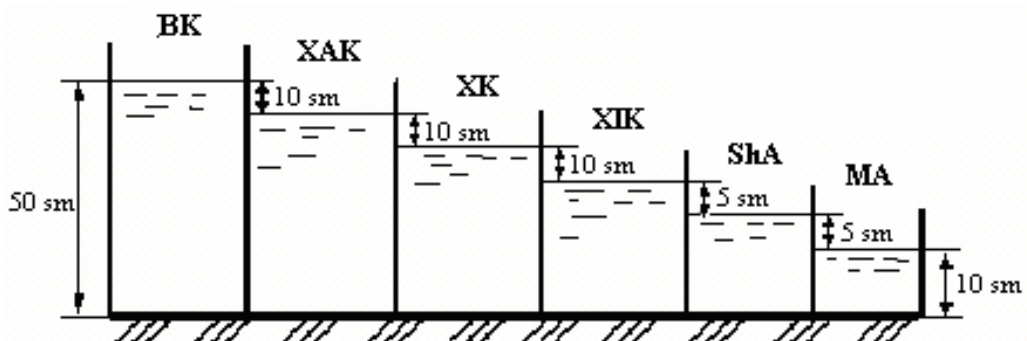
62-rasm. Sug‘orish tarmoqlarida suv sathi balandligini belgilash
