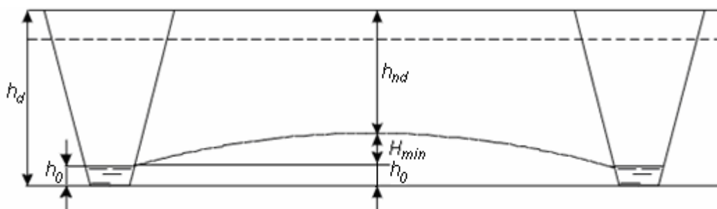
92-rasm. Sizot suvlari sathini gidrotexnik zovur yordamida pasaytirish
