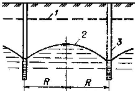
113-rasm. Tik zovurlar ta'sirida sizot suvlari sathining pasayishi sxemasi: 1, 2-sizot suvlarining oldingi va keyingi sathi; 3- burg'u qudug'i; R - burg'u qudug'ining ta'sir radiusi
