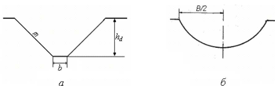
116-rasm. Kollektorlarning ko‘ndalang kesim ko‘rinishlari: a -trapetsiya shakli; b -parabola shakli
