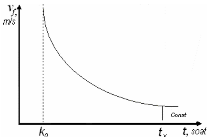
9-rasm. Suvning tuproqqa shimilish qonuniyati
