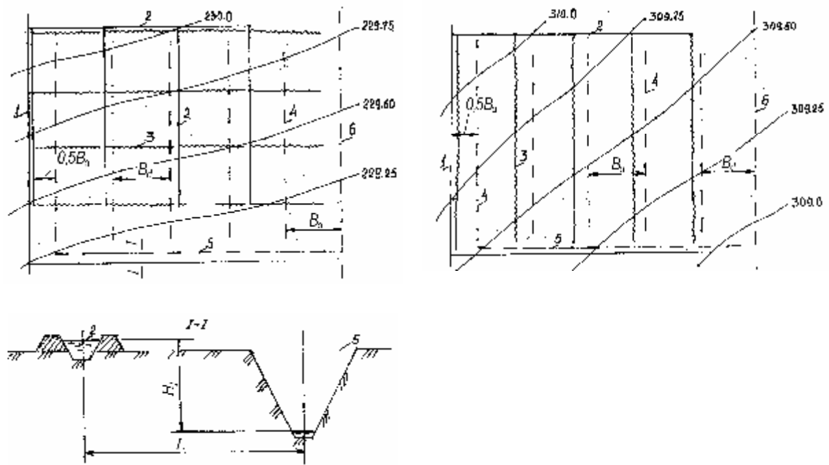
108-rasm. Yotiq zovurlarni rejada joylashtirish sxemasi
