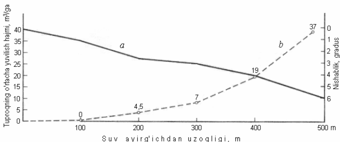
128-rasm. Qavariq yonbag'ir nishabligi va suv ayirg'ichdan uzoqligi bo'yicha qumoq tuproqlarning yuvilish hajmi
