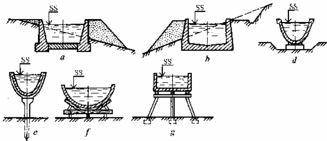
63-rasm. Novli sug'orish tizimlari: a -trapetsiya shaklida; b,g -to'rtburchak shaklida; d,e -parabola shaklida; f -yarim aylana shaklida
