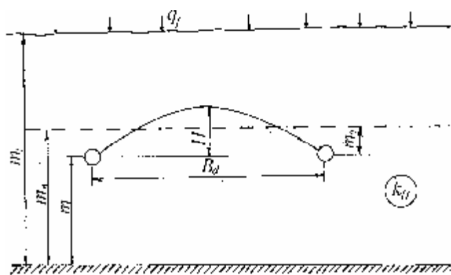
103-rasm. Suv o'tkazmaydigan qatlamga tiralgan 1 tarkibli qatlam
