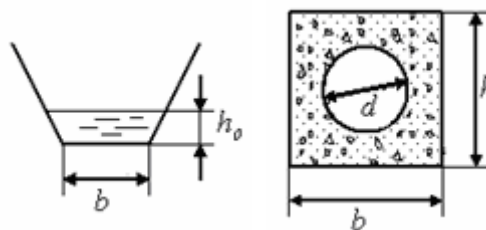
104-rasm. « d_x » ni aniqlash sxemasi
