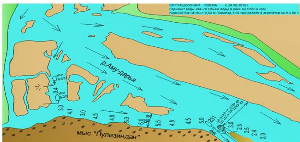
Рис.6 Ситуационная схема бесплотинного водозабора КМК
