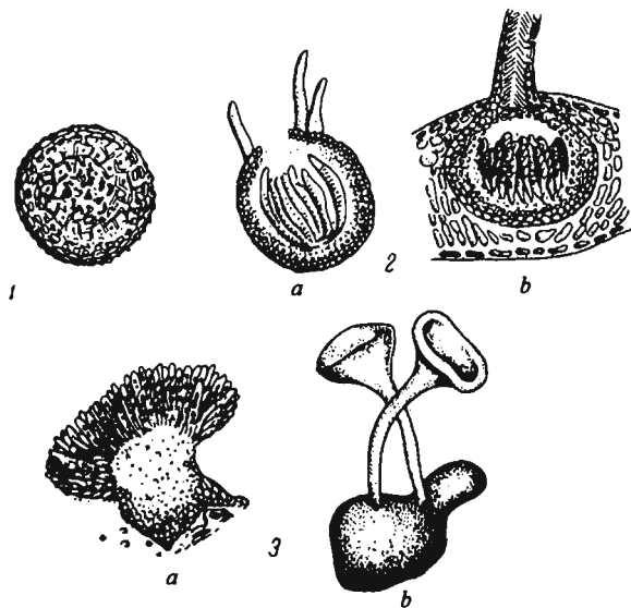
11-rasm. Xaltachali zamburug'larining mevtanalari:
