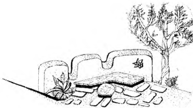
7.6-rasm. Manzarali dam olish joylarini chizmada tasvirlash.
