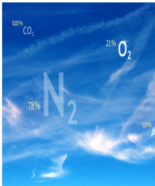
5-rasm. Atmosfera va uning tarkibiy tuzilishi
