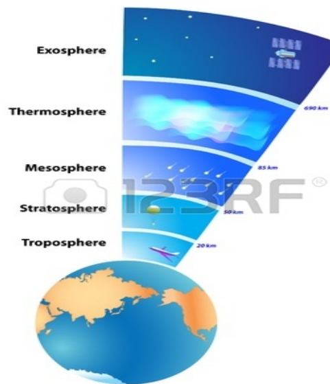
5-rasm. Atmosfera va uning tarkibiy tuzilishi
