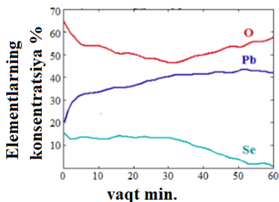
2-rasm. XPS ma'lumotlari bo'yicha Se, O, Pb elementlarning PbSe plyonkasi chuqurligi bo'yicha taqsimlanishi. tezligi ~6 nm/min.
