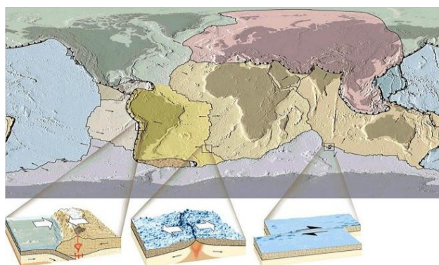
2-rasm. Litosfera plitalarining turli qismlaridagi deformatsiyalar
