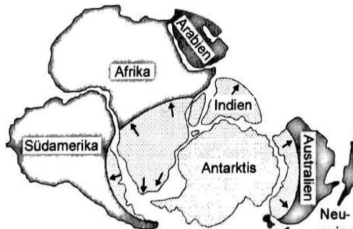
4-rasm. Mobilizm gipotezasiga muvofiq tuzilgan geotektura: Pangeya va Pantalassa
