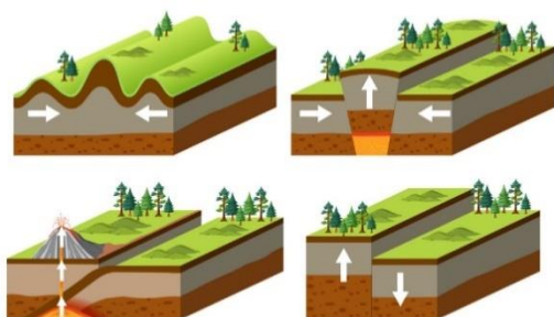
1-rasm. Tektonik harakatlarning turli ko'rinishlari
