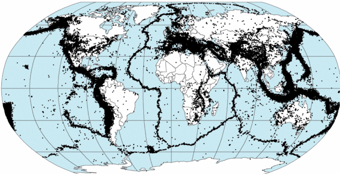
3-rasm. Zilzila tez-tez takrorlanib turadigan eng asosiy nuqtalar
