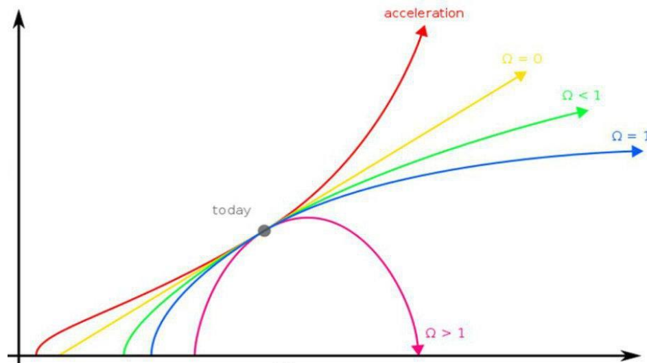
1-rasm. Kosmik kengayish dinamikasi
